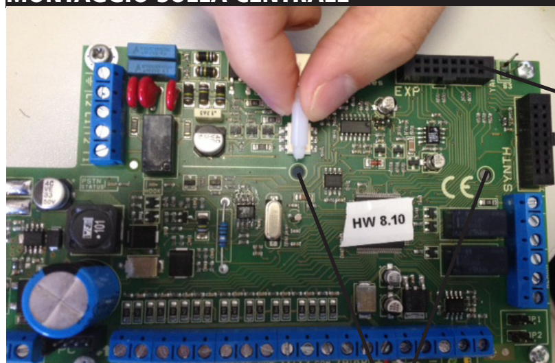
fori perni di fissaggio
