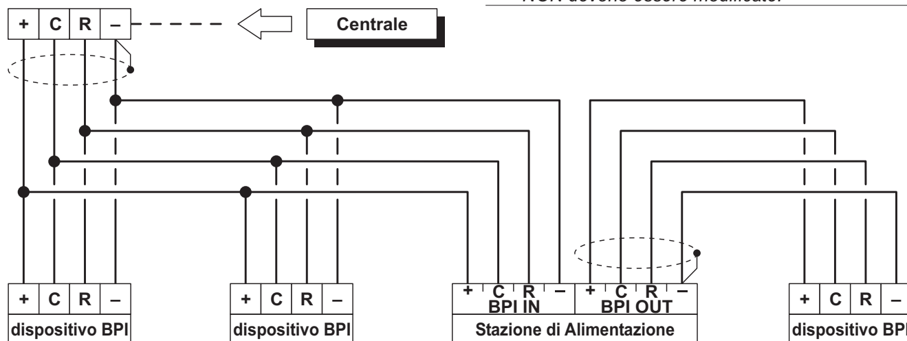
Figura 9 Collegamento di 4 Dispositivi BPI
