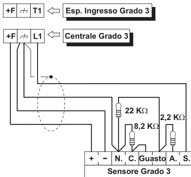
Figura 14 Collegamento di un sensore ad una zona con Bilanciamento Fine Linea Triplo .
