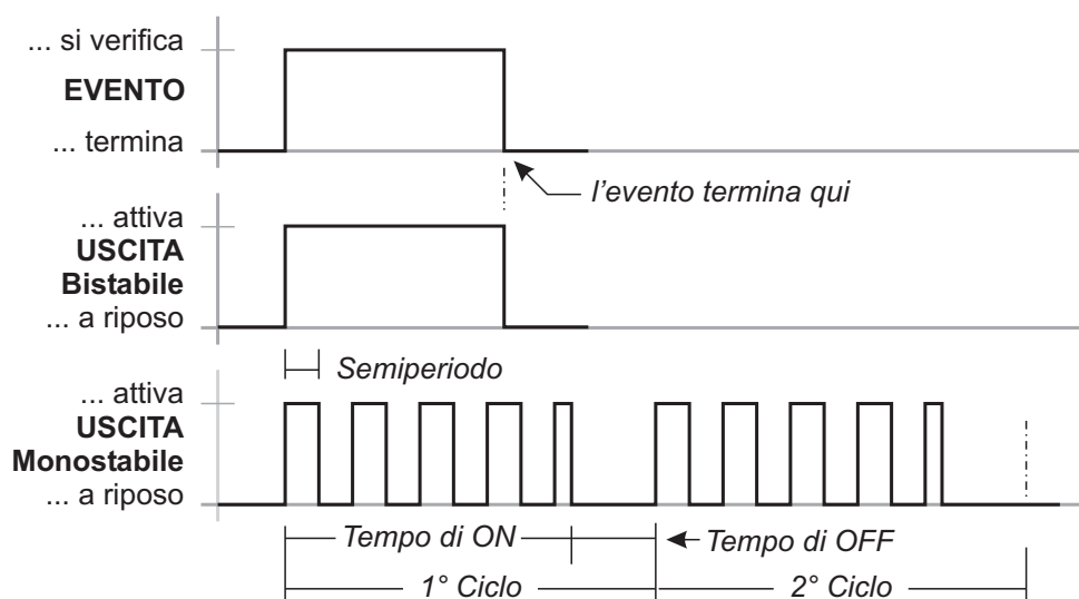
Figura 28 Effetto delle opzioni Semiperiodo e Cicli sulle Uscite Bistabile e Monostabile.
