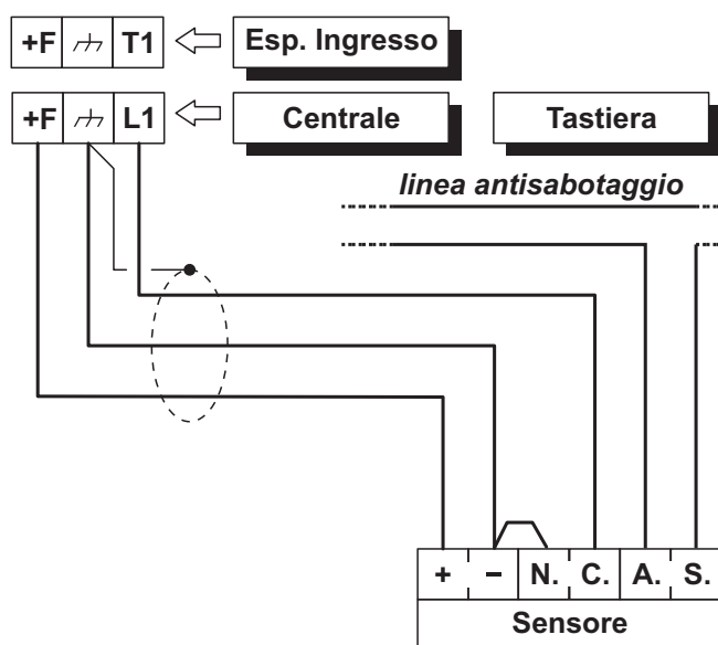
Figura 11 Collegamento di un sensore ad una zona con Bilanciamento Normalmente Chiuso.
