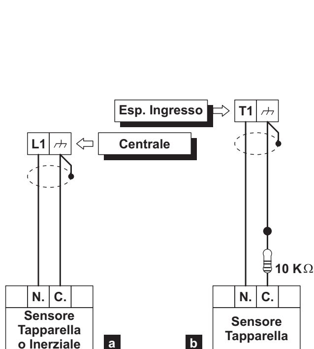
Figura 16 Collegamento di sensori inerziali (solo per le zone della centrale) e contatti per tapparella: collegamento di un sensore ad una zona con Bilanciamento Normalmente Chiuso (a), e di un sensore ad una zona con Bilanciamento Fine Linea Singolo (b).
