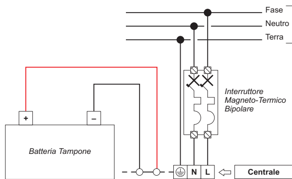
Figura 24 Collegamento dell'alimentazione.
