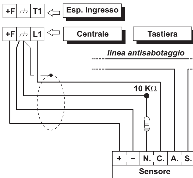
Figura 12 Collegamento di un sensore ad una zona con Bilanciamento Fine Linea Singolo.
