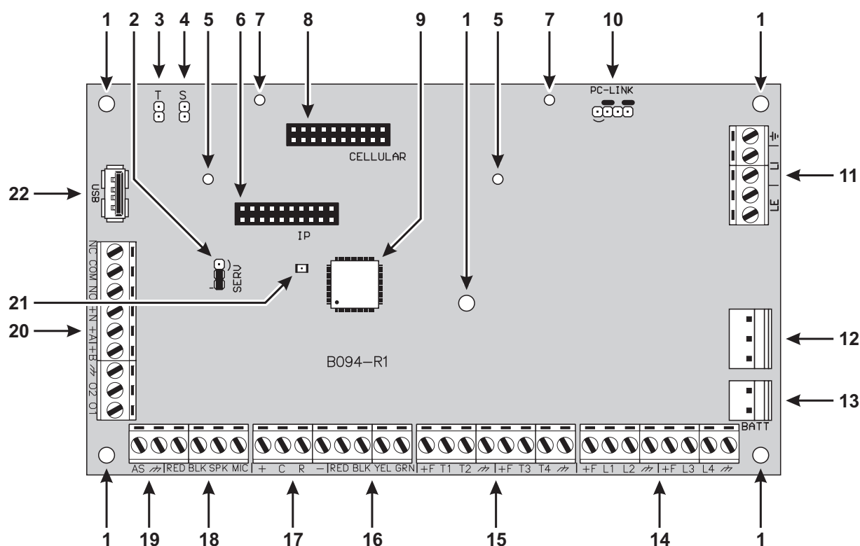
Figura 1 Scheda madre della centrale ABSOLUTA Plus.
