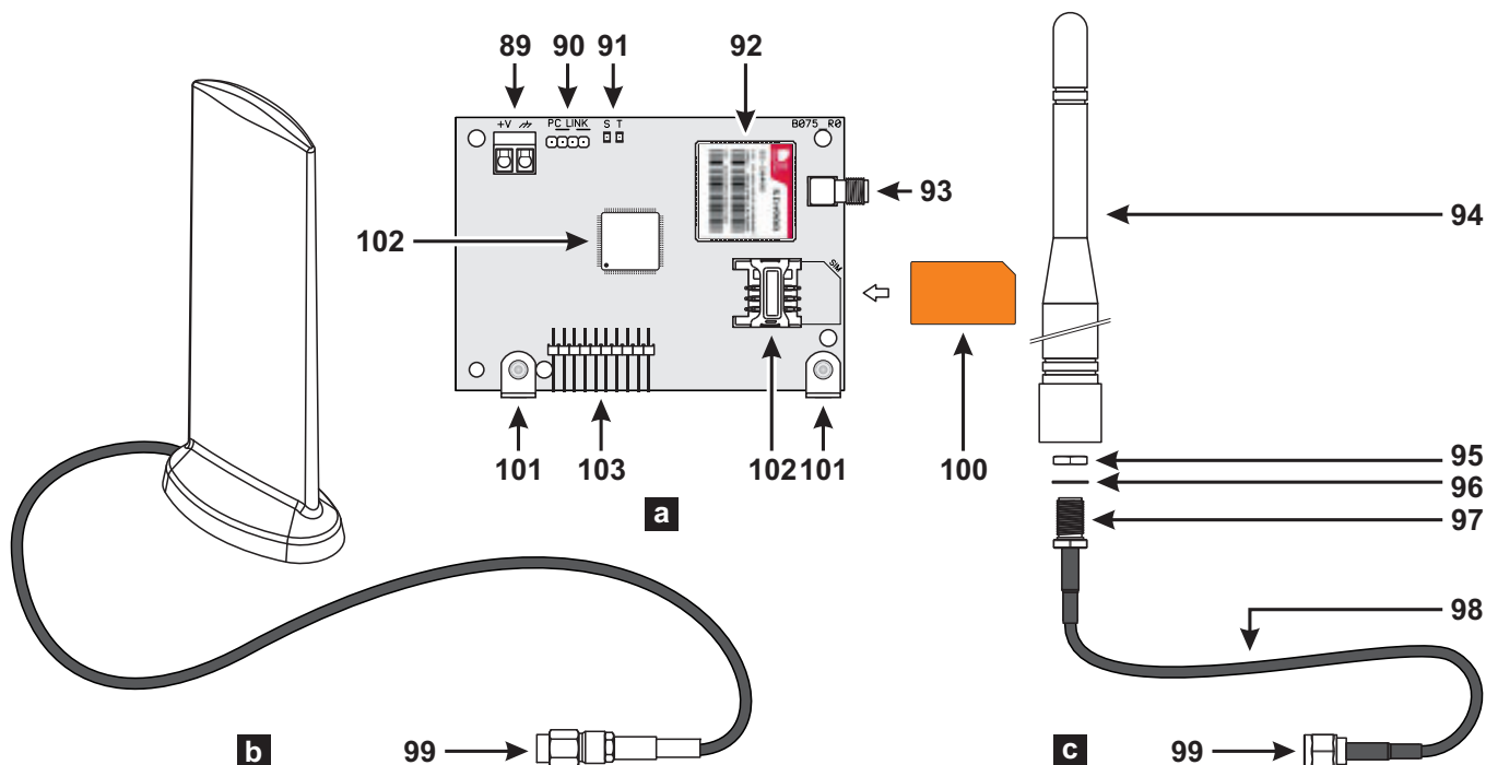
Figura 6 Parti del Modulo GSM ABS-GSM (a), dell'antenna per contenitore metallico ABS-AM (b), dell'antenna per contenitore plastico ABS-AK (c).
