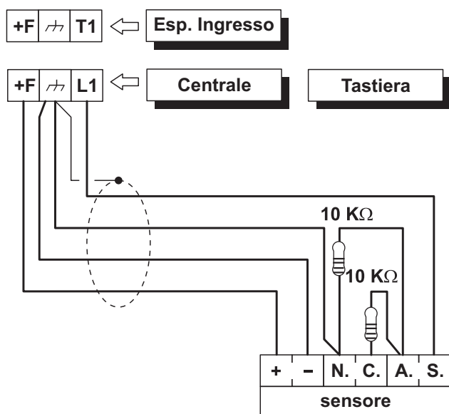
Figura 13 Collegamento di un sensore ad una zona con Bilanciamento Fine Linea Doppio .
