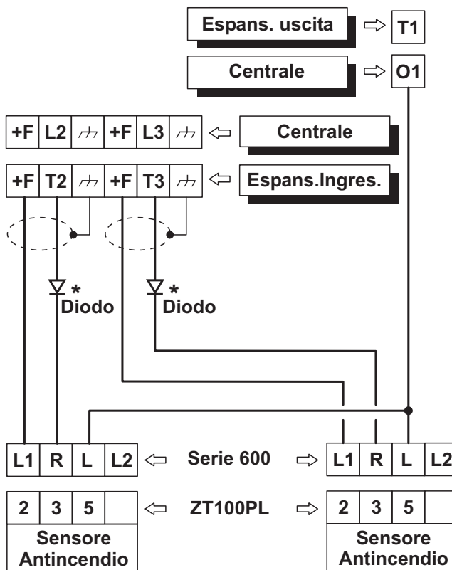
Figura 15 Collegamento di 2 sensori antincendio a Zona con Bilanciamento Normalmente Aperto (* Solo con la serie 600).
