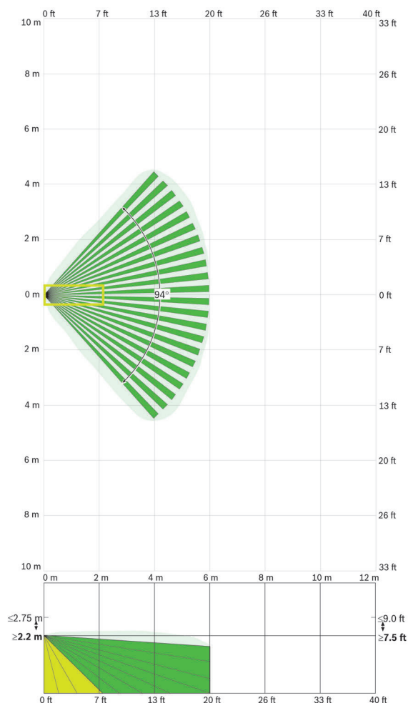
Copertura 6 m x 6 m (ISC-BDL2-WP6G, ISC-BDL2-WP6G-CHI)
