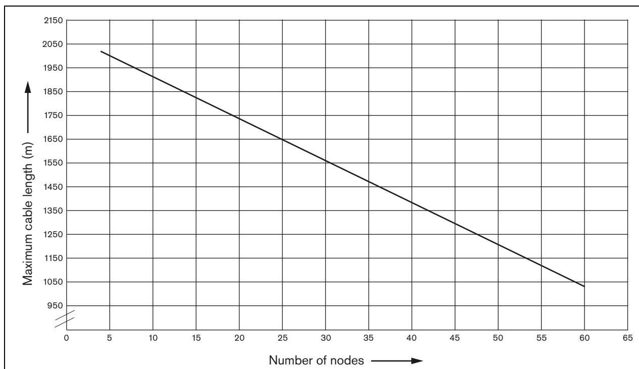
figura 20.5: Lunghezza massima delle fibre ottiche contro numero di nodi
