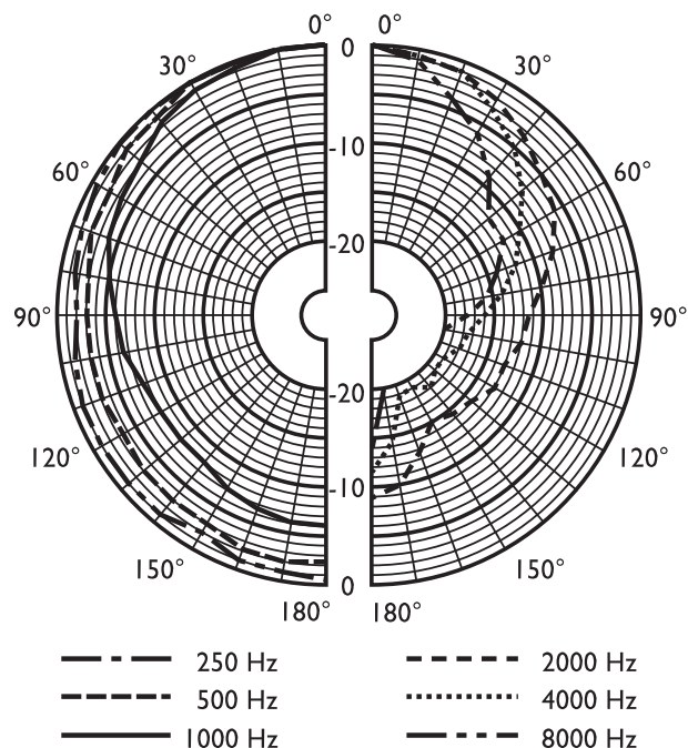
Diagramma polare (misurato con il rumore rosa)
