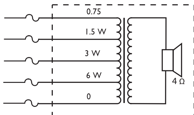
Diagramma del circuito
