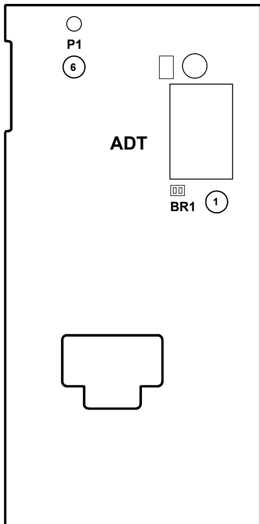
Lato saldato:
