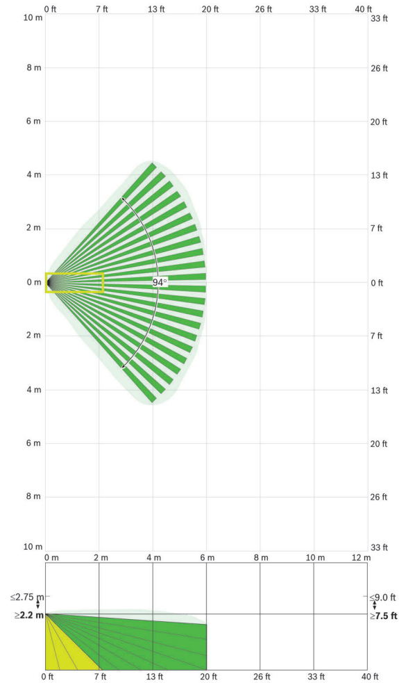
Copertura 6 m x 6 m (ISC-BDL2-WP6G, ISC-BDL2-WP6G-CHI)
