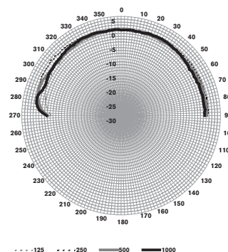
LC1-UM12E8 risposta in frequenza
