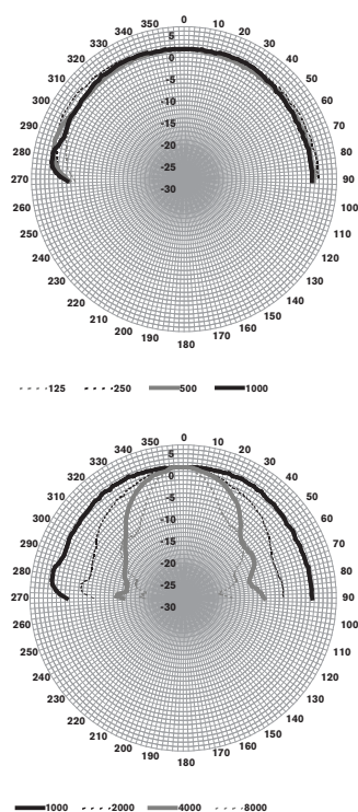
Figure polari di LC1-UM06E8
