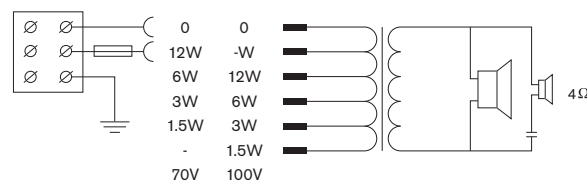
Schema circuitale di LC1-UM12E8
