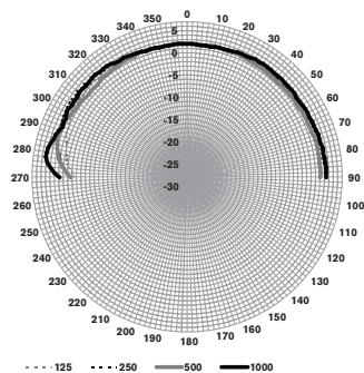
LC1-WC06E8 risposta in frequenza
