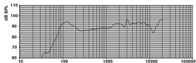
LC1-UM06E8 risposta in frequenza
