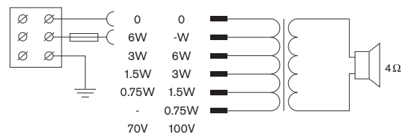
Schema circuitale di LC1-WM06E8
