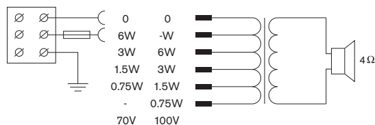
Schema circuitale di LC1-WC06E8
