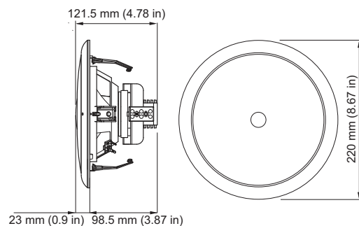
Dimensioni in mm di LC1-UM12E8
