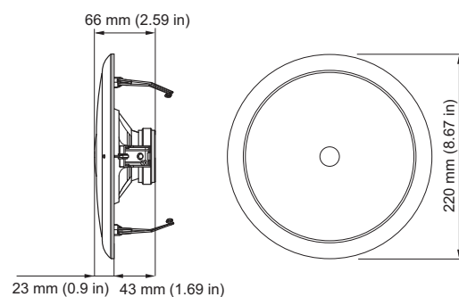
Dimensioni in mm di LC1-WM06E8
