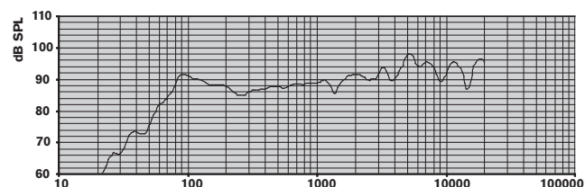
LC1-UM12E8 risposta in frequenza
