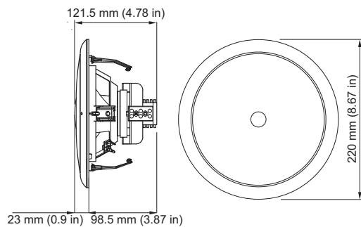
Dimensioni in mm di LC1-UM24E8
