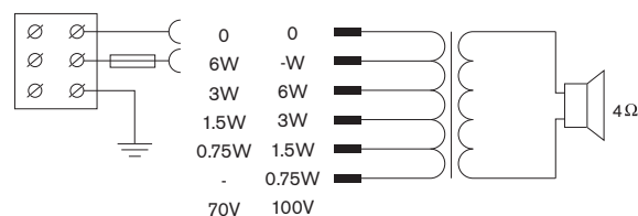
Schema circuitale di LC1-UM06E8
