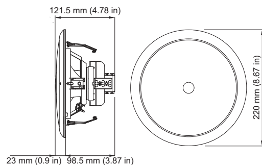
Dimensioni in mm di LC1-UM06E8
