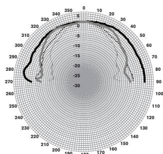
Figure polari di LC1-WM06E8
