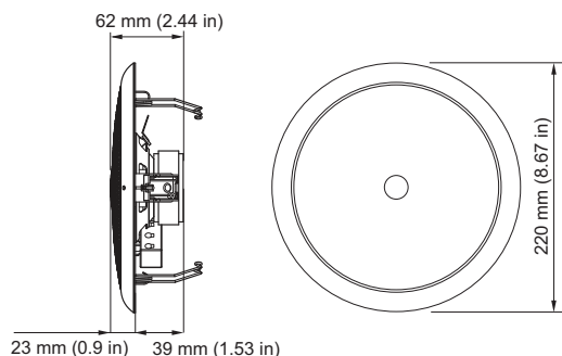
Dimensioni in mm di LC1-WC06E8
