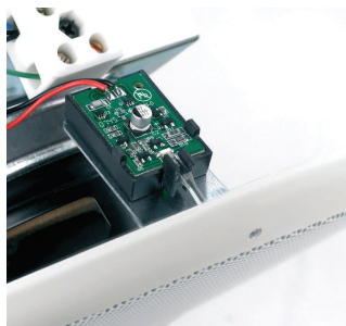
LC1-PIB installata sull'altoparlante ed indicante il conduttore luminoso
