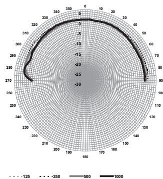
LC1-UM24E8 risposta in frequenza
