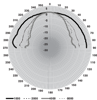
Figure polari di LC1-WC06E8
