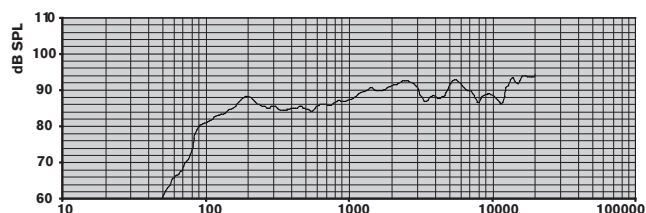
LC1-WM06E8 risposta in frequenza
