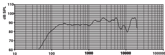
LC1-WC06E8 risposta in frequenza
