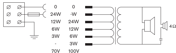
Schema circuitale di LC1-UM24E8
