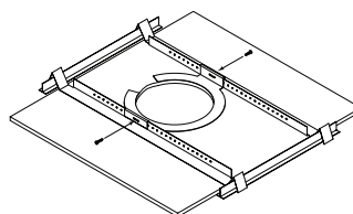
LM1-TB telaio per controsoffittatura/guarnizione C-Ring
