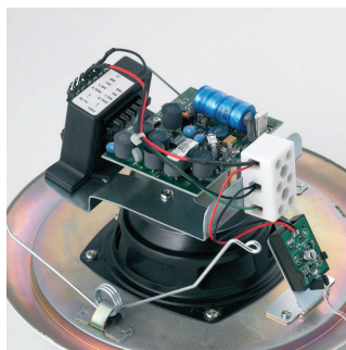
Vista posteriore di LC1-WM06E8 in cui sono mostrati il montaggio opzionale per LC1-PIB e la scheda di sorveglianza linea/altoparlanti opzionale
