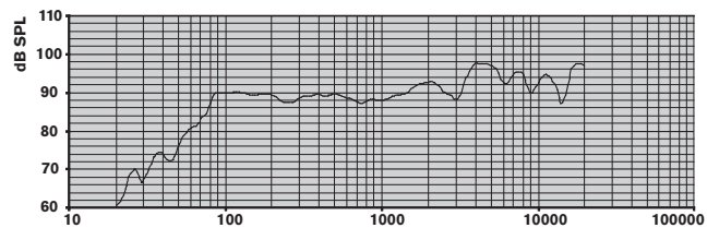
LC1-UM24E8 risposta in frequenza
