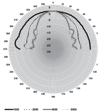
Figure polari di LC1-UM24E8
