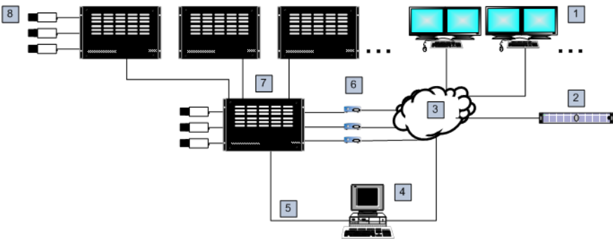
Figura 5.5: Sistema Bosch Allegiant esteso con commutatori satellitari
