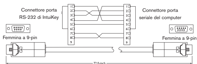
FIGURA 2-8 Piedinatura del cavo S1385
