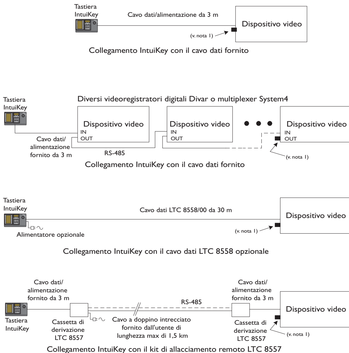
FIGURA 2-4 Opzioni di collegamento tipiche per IntuiKey
