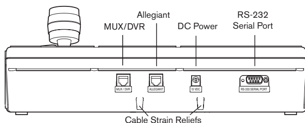
FIGURE 2-2 Pannello posteriore della tastiera IntuiKey
