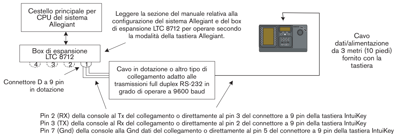
FIGURA 2-6: Configurazione mediante box di espansione porta Console LTC 8712
