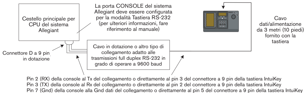
FIGURA 2-5: Collegamento diretto alla console Allegiant e alla porta Printer
