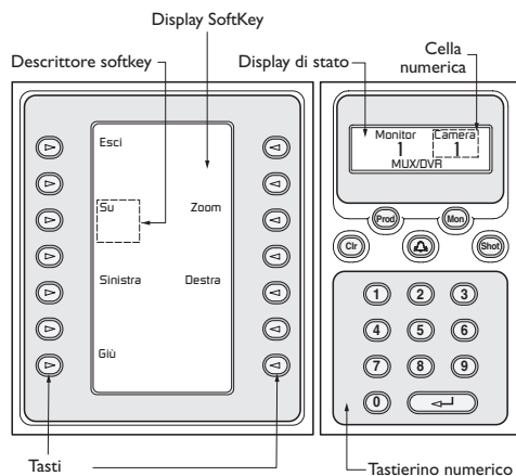
FIGURA 3-1 Componenti della tastiera Intuikey
