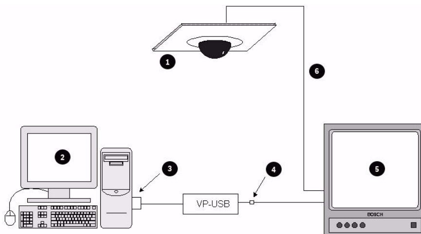
Immagine 3.1 Collegamento del Tool di Configurazione VP-USB
