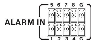
Immagine 4.12 Connettore di ingresso allarme per il modello a 8 canali
