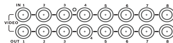
Immagine 4.2 8 ingressi video con uscite loop-through
