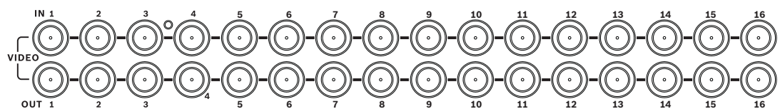
Immagine 4.1 16 ingressi video con uscite loop-through
