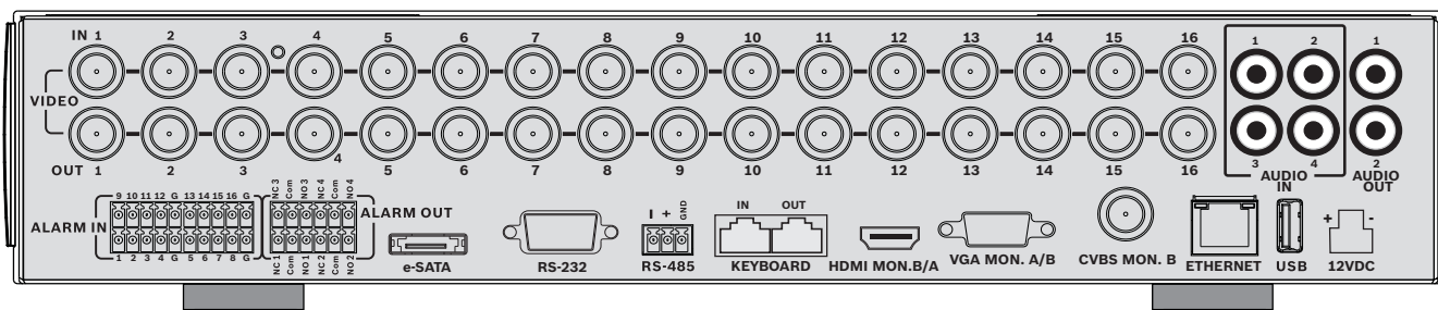
Immagine 3.1 Collegamenti del pannello posteriore per il modello a 16 canali
