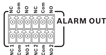
Immagine 4.13 Connettore di uscita allarme
