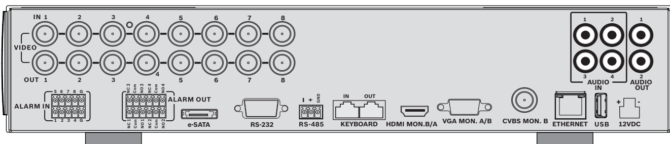
Immagine 3.2 Collegamenti del pannello posteriore per il modello a 8 canali
