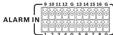
Immagine 4.11 Connettore di ingresso allarme per il modello a 16 canali
