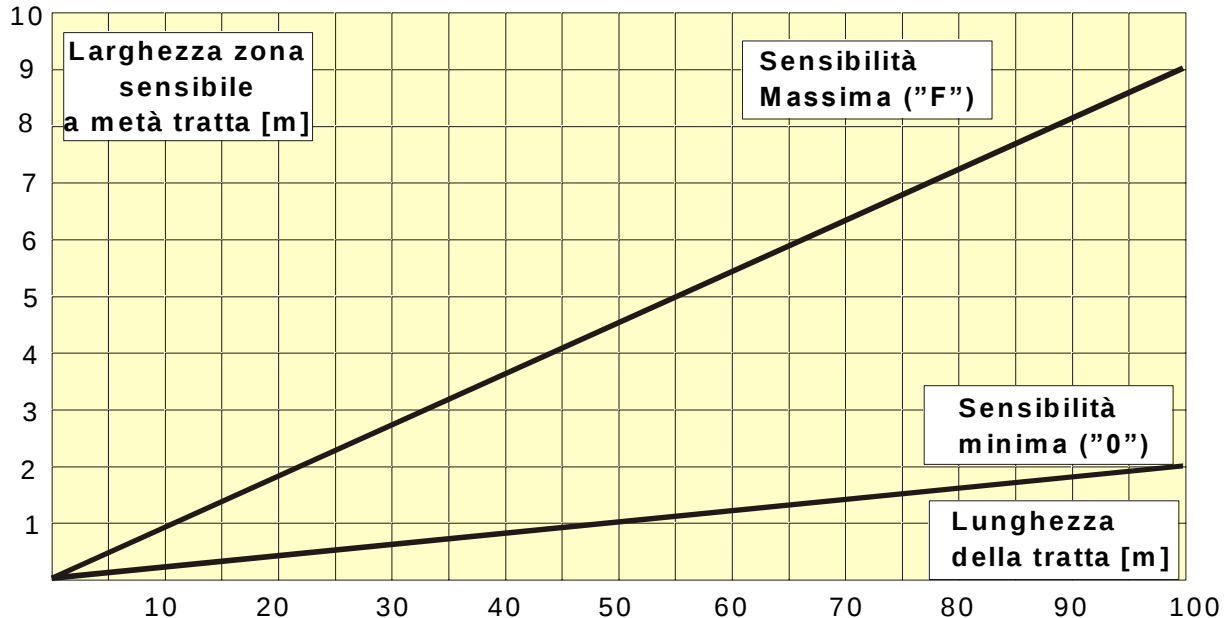
Figura 3 Larghezza della zona sensibile a metà tratta per CORAL 100 sul piano orizzontale (campo libero)
