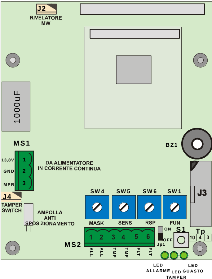
Figura 9 Disposizione topografica dei componenti nel circuito Rx
