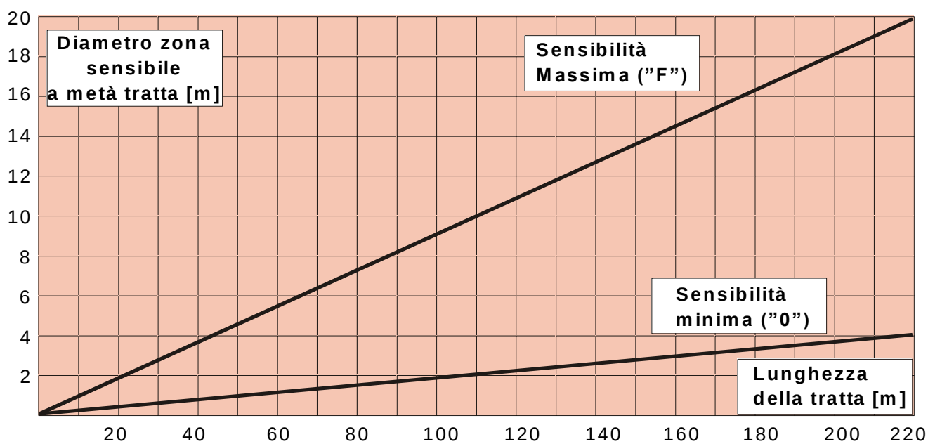
Figura 4 Diametro della zona sensibile a metà tratta per CORAL-220 (campo libero)
