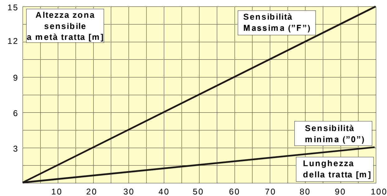
Figura 3a Altezza della zona sensibile a metà tratta per CORAL 100 sul piano verticale (campo libero)
