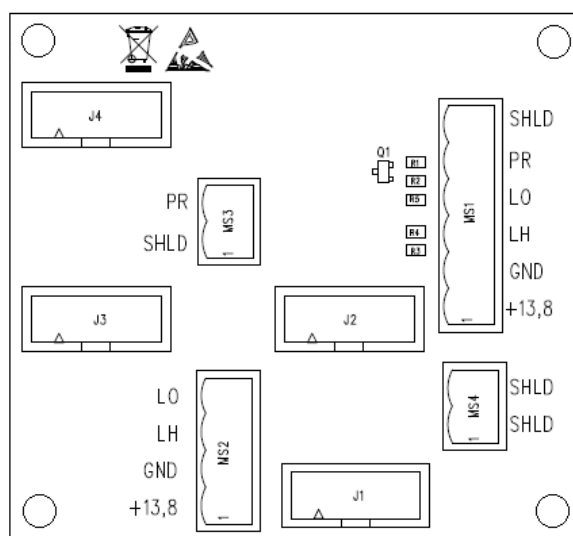
Figura 13 Disposizione topografica dei componenti nel circuito
