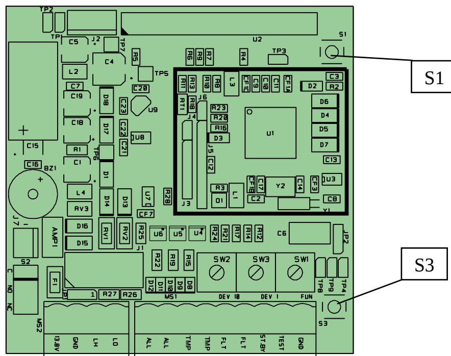
Figura 12 Disposizione topografica dei componenti nel circuito
