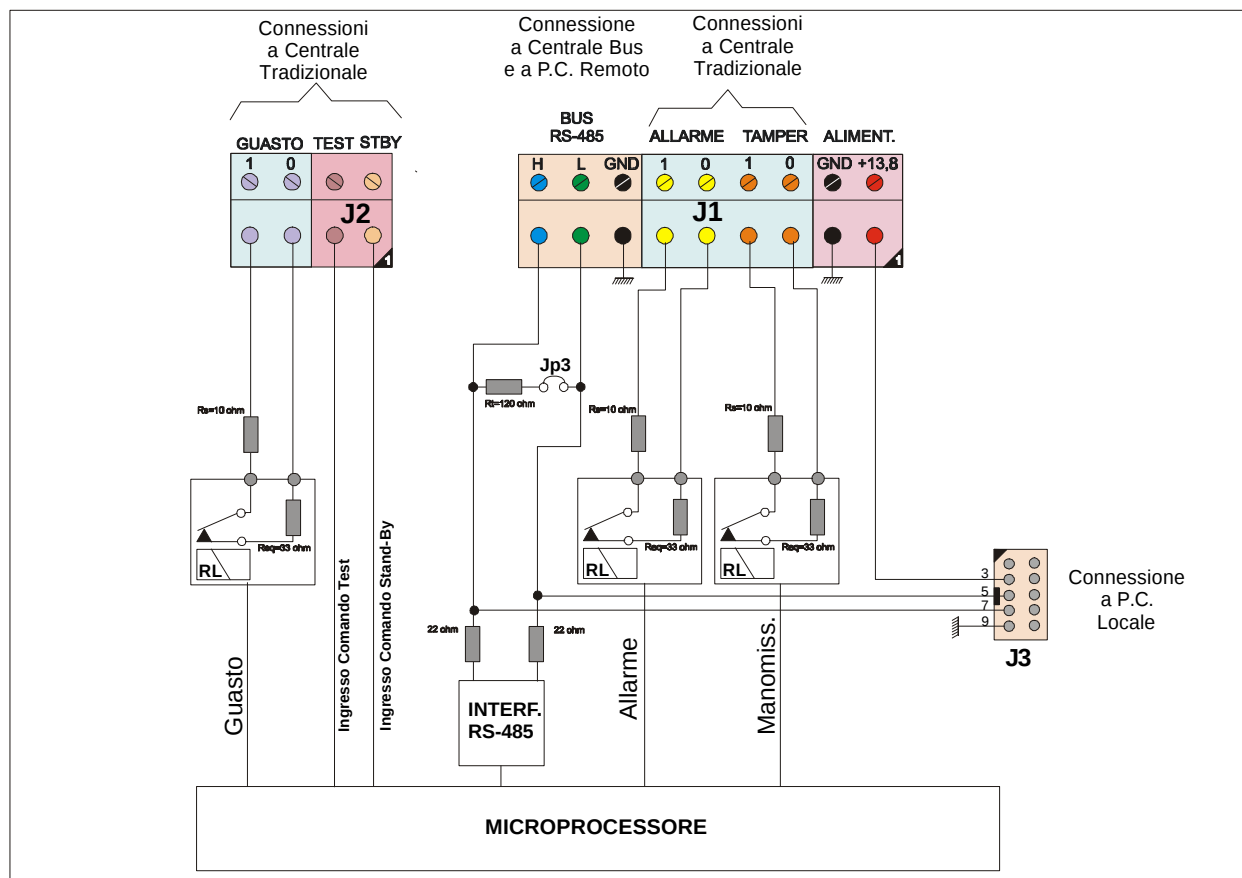
Schema morsettiere J1 e J2
