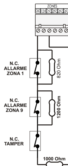
CONTATTO N.C. DI ALLARME ZONA 1, CONTATTO N.C. DI ALLARME ZONA 9 E CONTATTO N.C. DI TAMPER CON RESISTENZE DI TRIPLO BILANCIAMENTO
