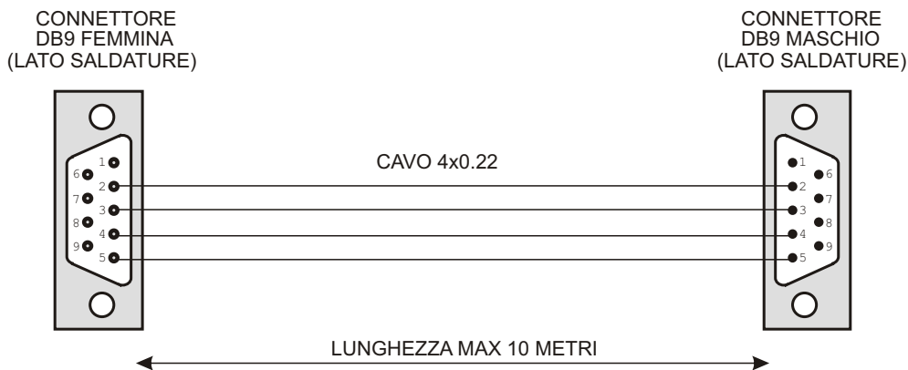
Figura 1.bis: schema di cablaggio cavo di programmazione RS232 per Amica 64 Plus 2009.
