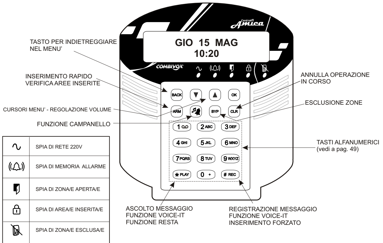
Figura 2 : riepilogo tasti e indicazioni luminose della tastiera (vedi a pag. 48).
