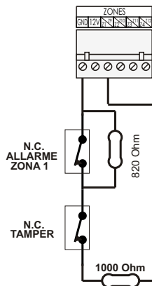
CONTATTO N.C. DI ALLARME E CONTATTO N.C. DI TAMPER CON RESISTENZE DI DOPPIO BILANCIAMENTO
