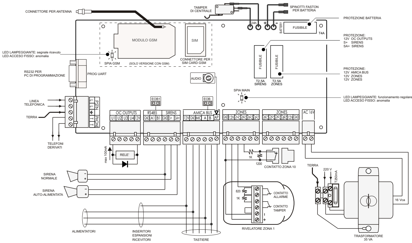
Figura 1: Schema di cablaggio Amica 64 Plus 2009.
