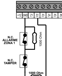
CONTATTO N.C. DI ALLARME E CONTATTO N.C. DI TAMPÉR CON RESISTENZE DI DOPIO BILANCIAMENTO
