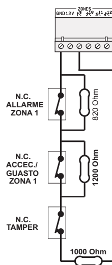
CONTATTO N.C. DI ALLARME ZONA 1, CONTATTO N.C. DI ACCECCAMENTO/GUAUSTO ZONA 1 E CONTATTO N.C. DI TAMPER CON RESISTENZE DI TRIPLO BILANCIAMENTO
