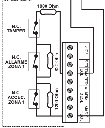
CONTATTO N.C. DI ALLARME ZONA 1, CONTATTO N.C. DI ACCECCAMENTO ZONA 1 E CONTATTO N.C. DI TAMPER CON RESISTENZE DI TRIPLO BILANCIAMENTO ALL'INTERNO DEL SENSORE
