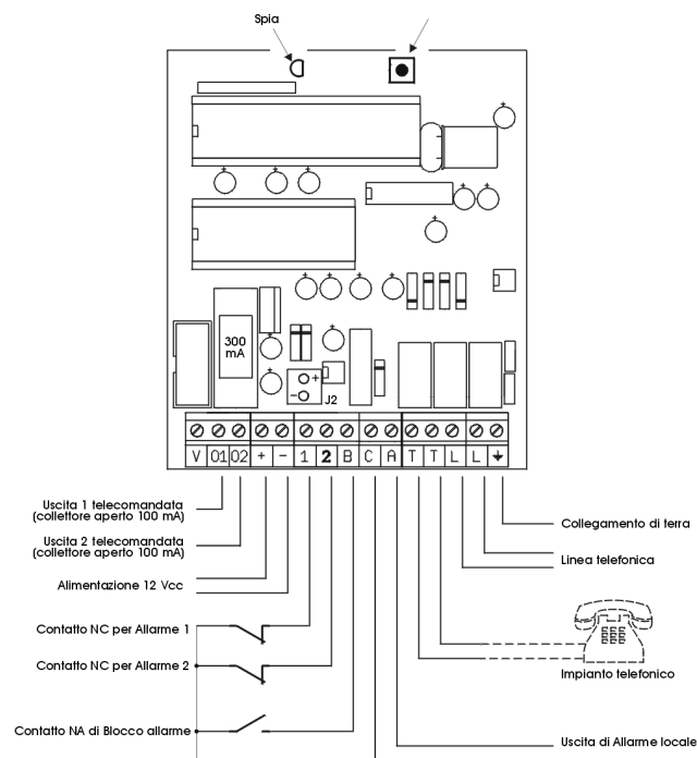
Figura 1 Collegamenti
