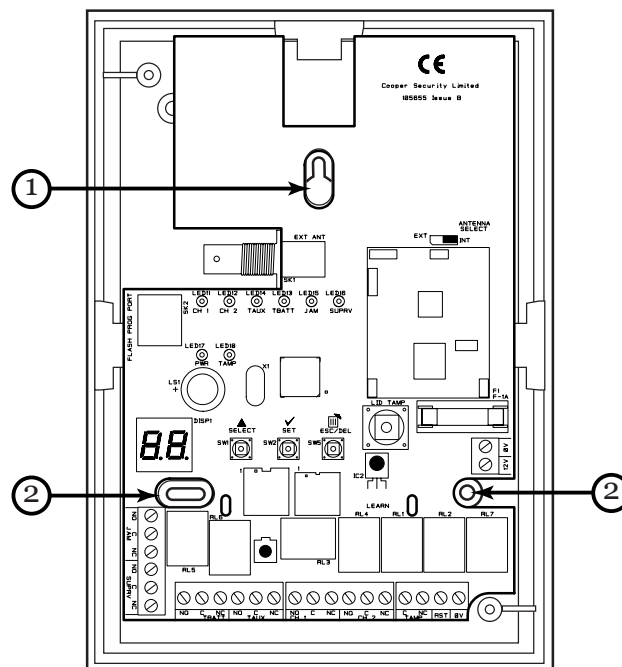
Figura 4. Posizioni dei fori di montaggio
