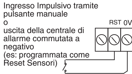
Figura 6. Collegamento Reset Esterno.
