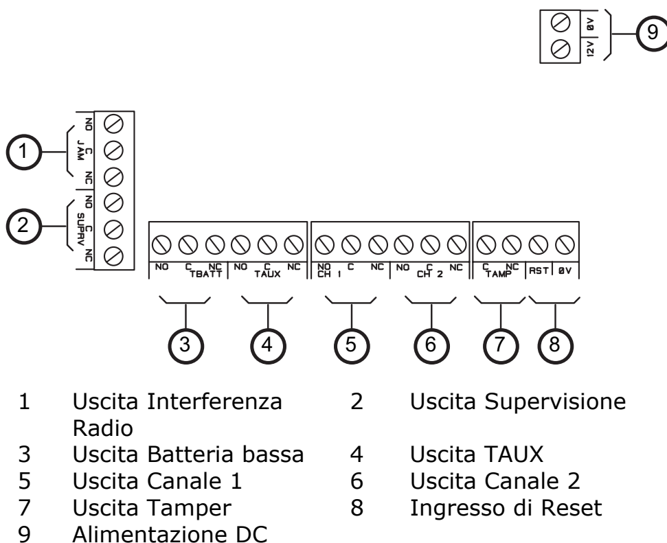
Figura 5. Connettore principale PCB.
