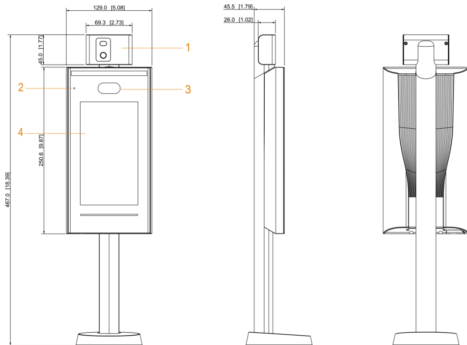
Figure 1-1 Dimensioni e componenti (mm [inch])
