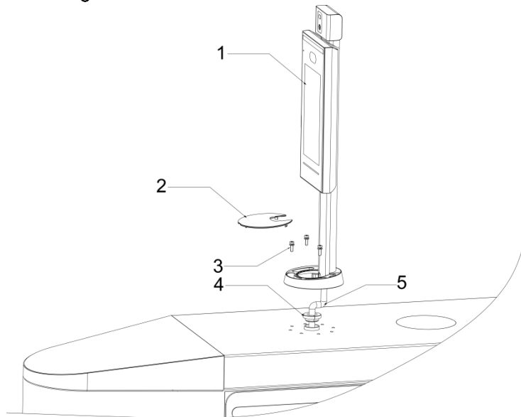
Figure 2-7 Applicare del sigillante siliconico al terminale
