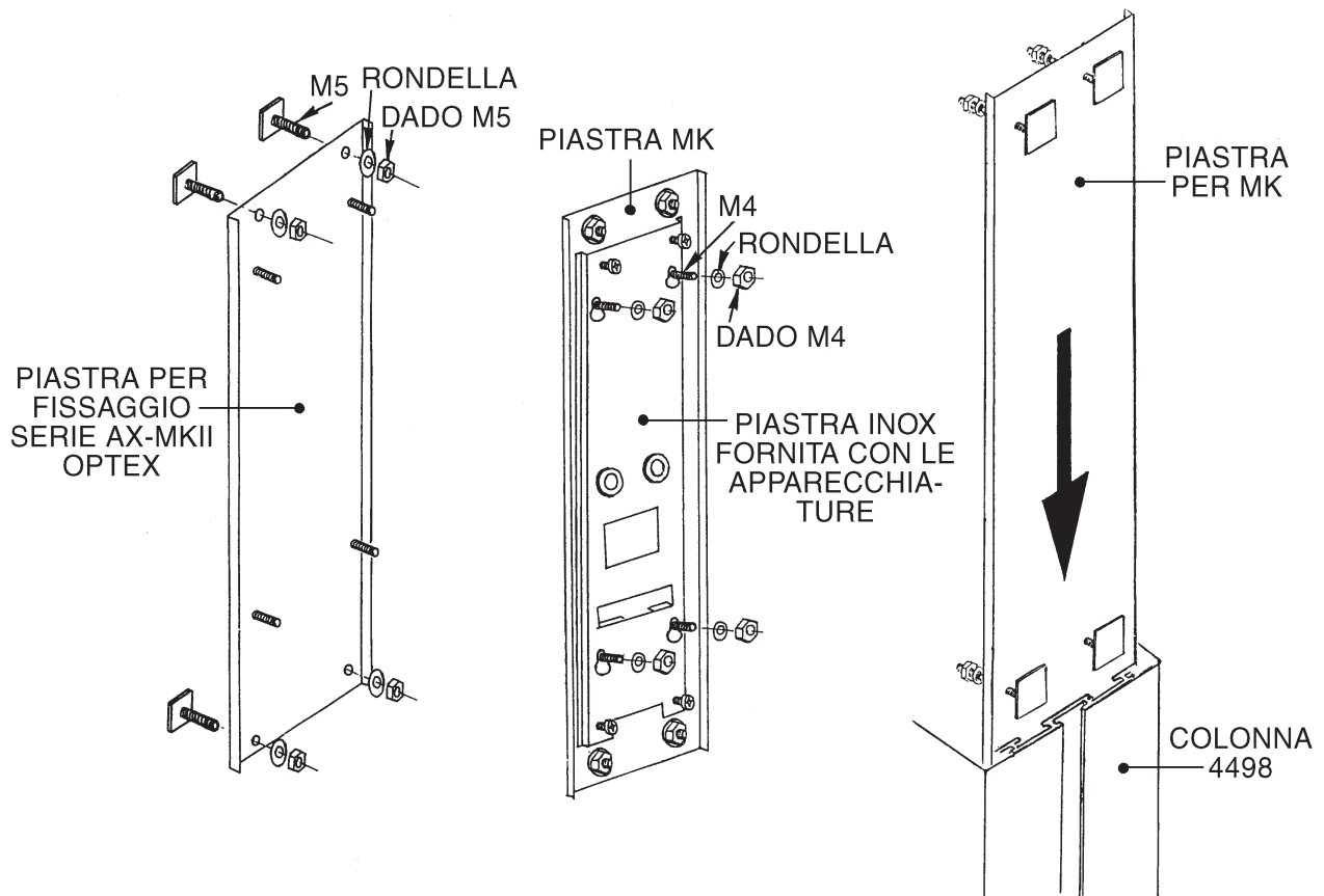
Schema di fissaggio piastra MK
