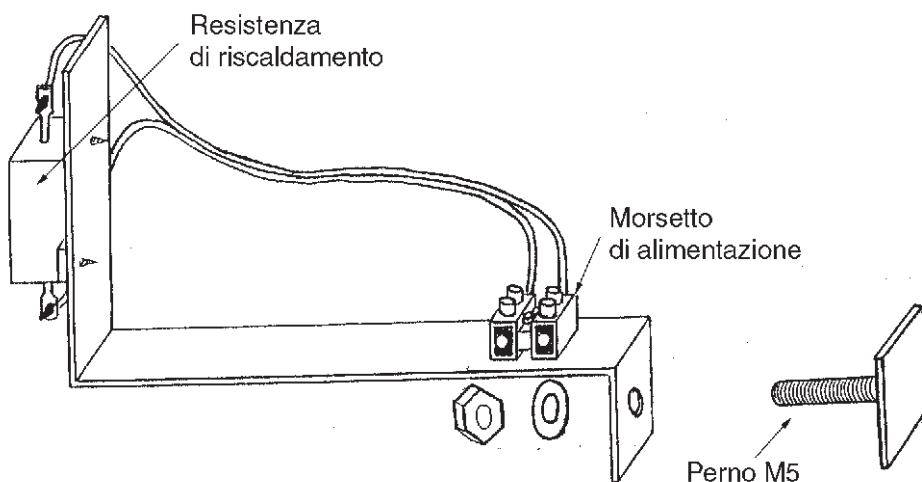
Figura 1 - Kit Riscaldatore art. 4498A
