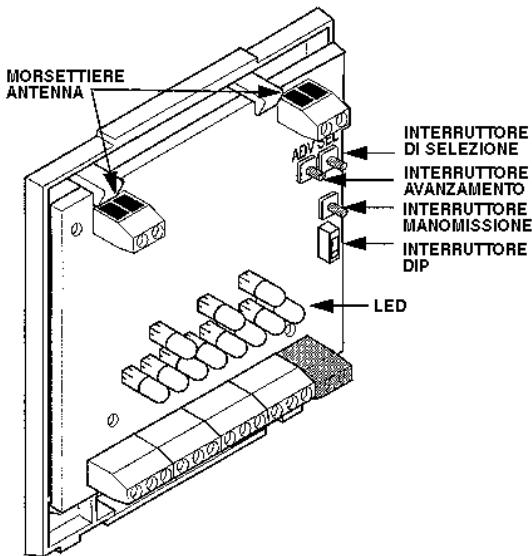
Fig. 1 - Componenti principali del Ricevitore
