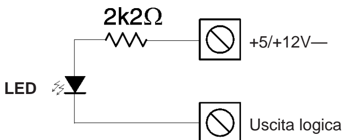
Accensione di un LED tramite un'uscita logica
