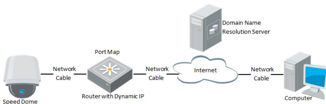
Figure 2-6 Risoluzione Normale del Nome del Dominio
