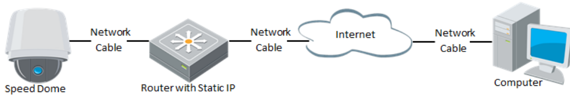
Figure 2-3 Accesso alla Speed Dome con un Router con IP Statico
