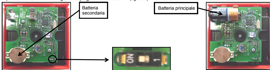
Figura 6 - la batteria secondaria e l'interruttore di collegamento-programmazione
