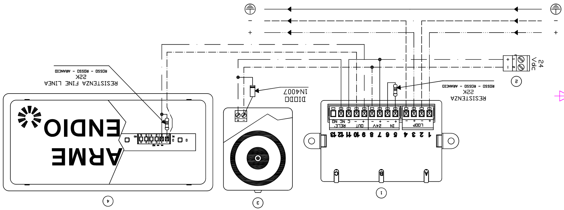
TIPICO COLLEGAMENTO USCITA MODULO EM312SR
