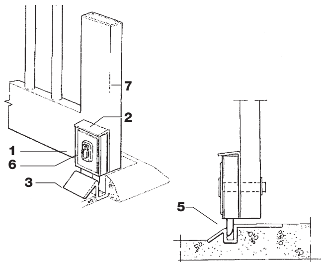
Mocowanie pionowe (dla dwóch skrzydeł)
