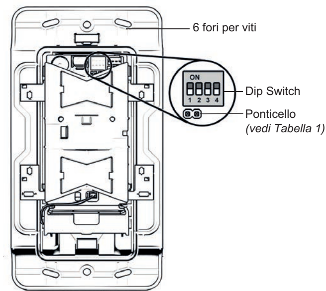
Figura 1: Vista Frontale – Coperchio Aperto
