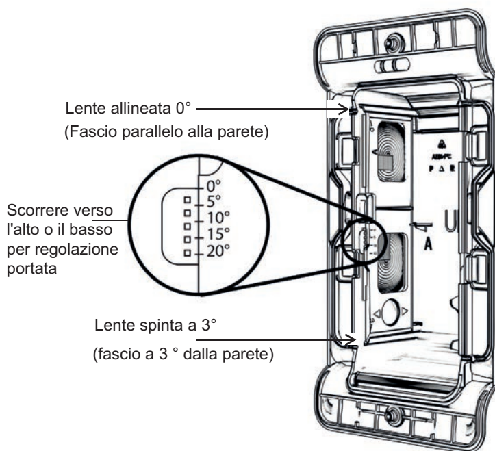
Figura 2: Fasci di rilevazione regolabili
