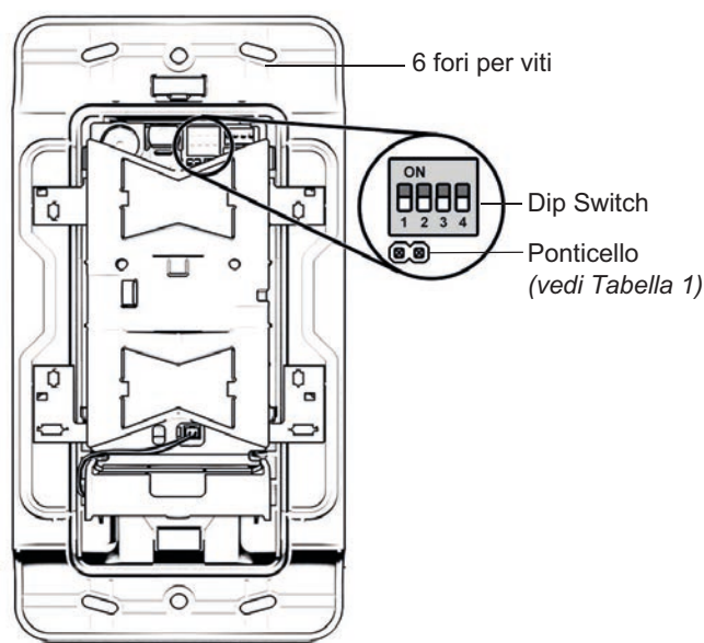
Figura 1: Vista Frontale – Coperchio Aperto
