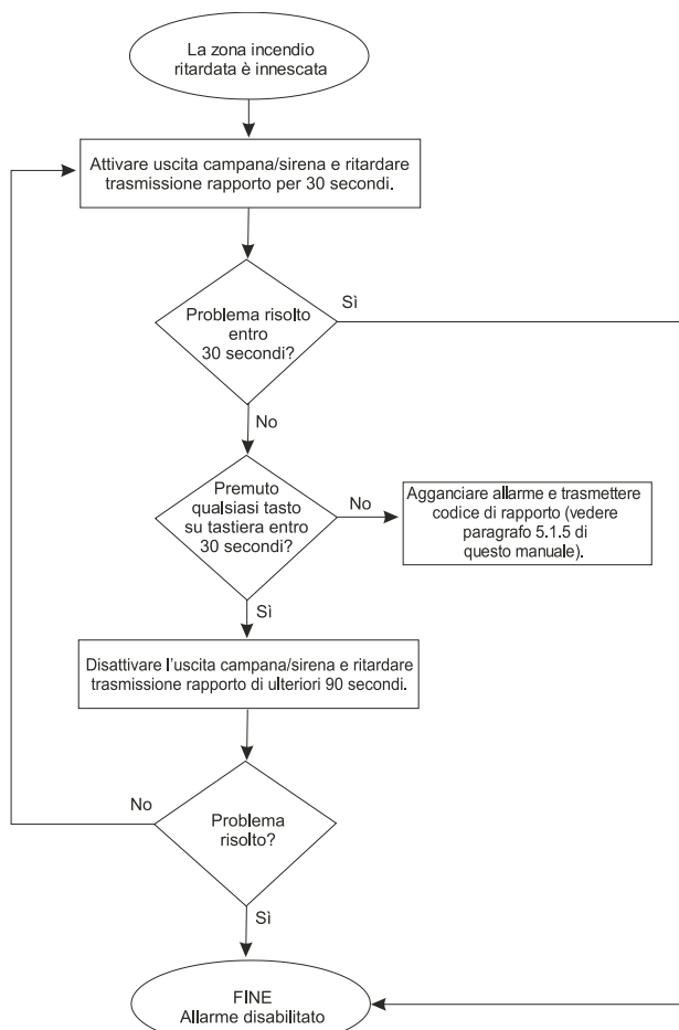
Figura 4-3: Zona incendio 24 ore ritardata
