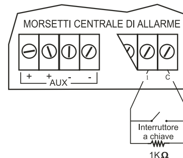
Figura 2-9: Connessioni interruttore a chiave
