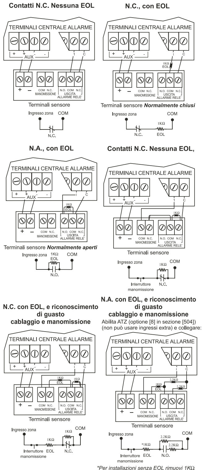
Figura 2-7: Connessioni ingressi zone singole
