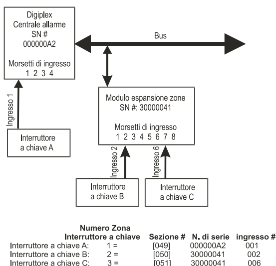
Figura 5-2: Esempio di numerazione di interruttori a chiave
