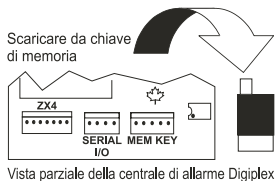
Figura 3-1: Uso della chiave di memoria
