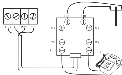
Figura 2-1 Connessioni linea telefonica
