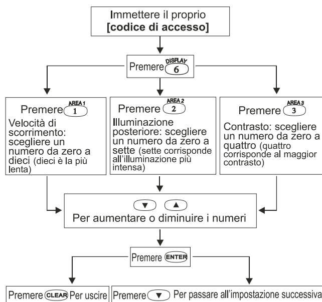
Figura 16-2: Impostazioni tastiera LCD
