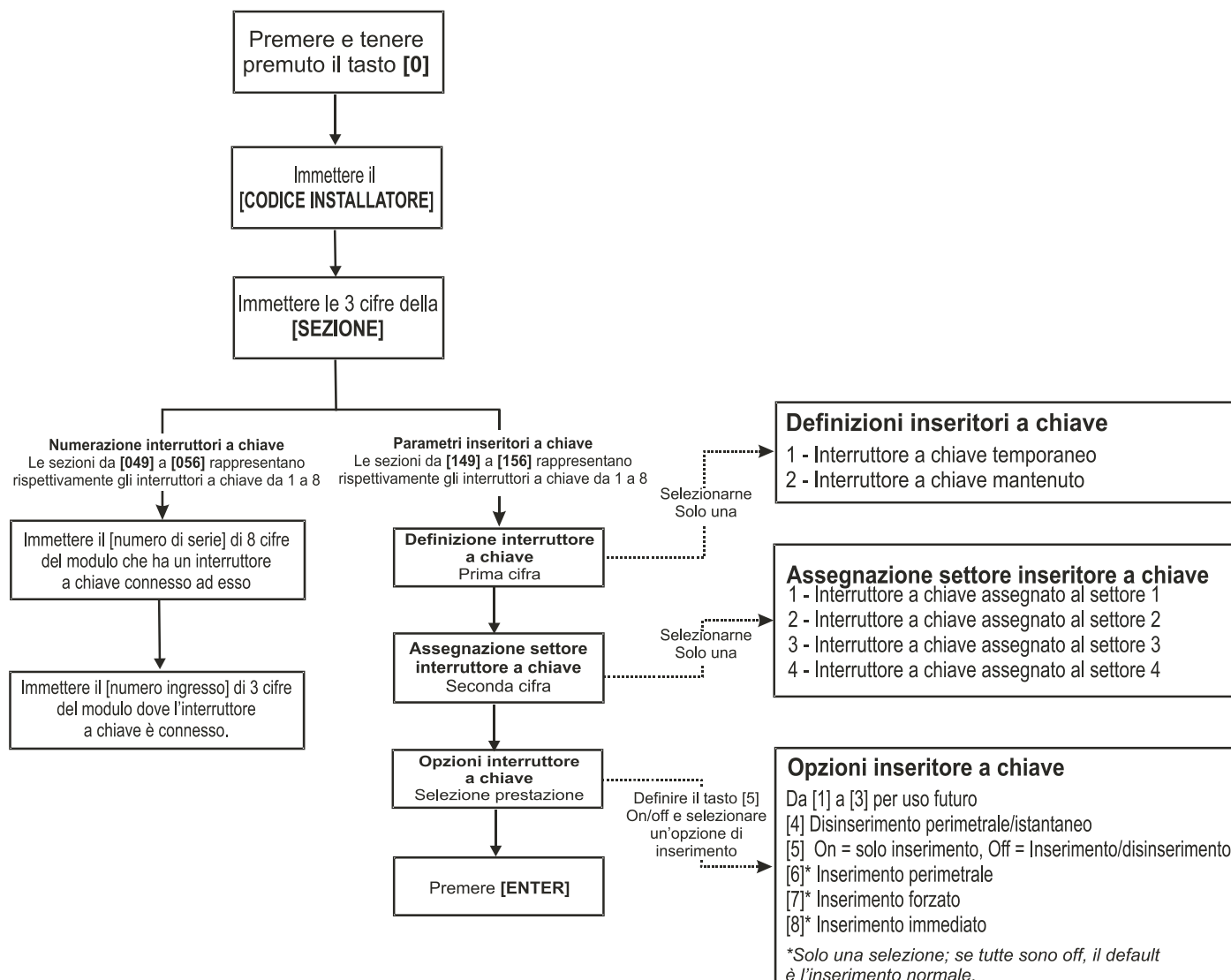
Figura 5-1: Programmazione inseritore a chiave
