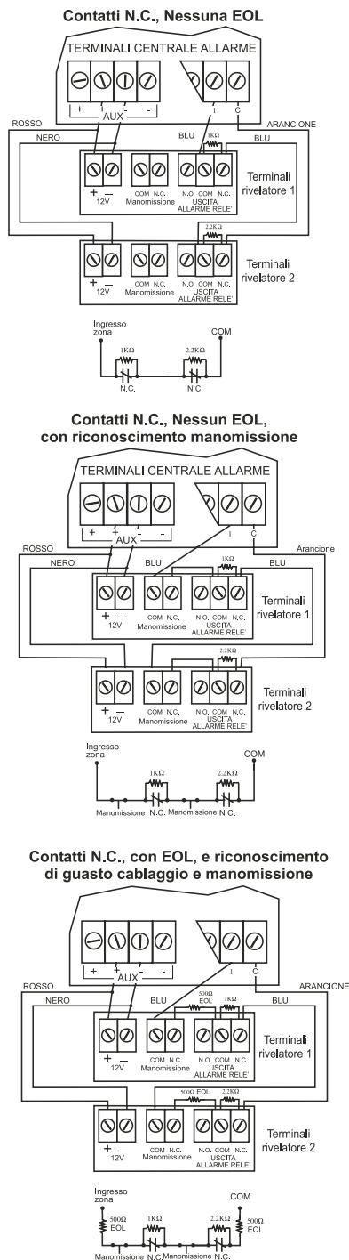
Figura 2-8: Connessioni di zone doppie
