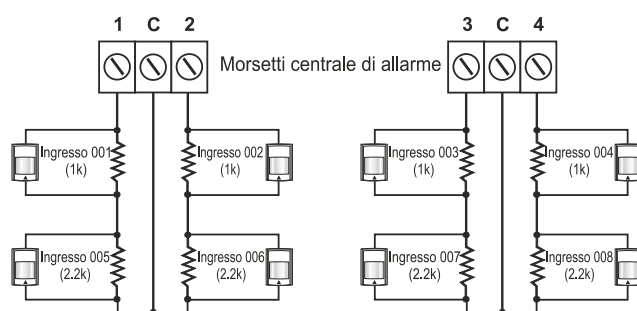
Figura 4-5: Riconoscimento morsetti ingresso ATX
