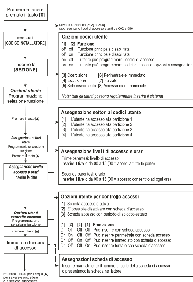
Figura 13-1: Programmazione codici accesso utente
