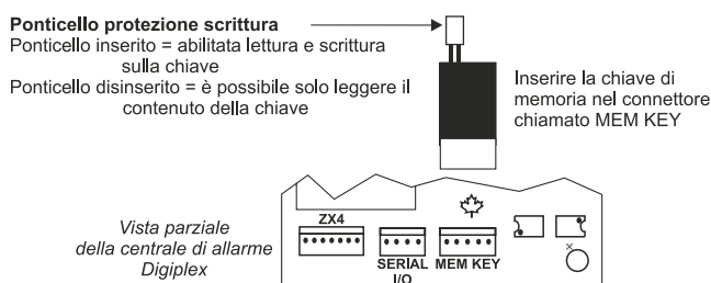
Figura 3-1: Uso della chiave di memoria
