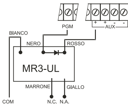
Figura 2-6: Uscita relè PGM
