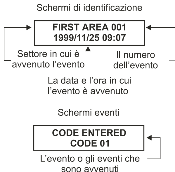
Figura 16-3: Schermi registro eventi
