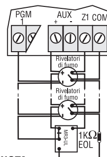
Figura 9: rivelatori a 4 fili
