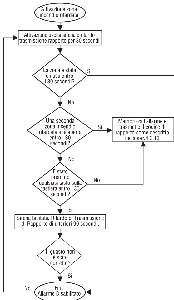
Figura 13: Zona incendio 24 ore ritardata
