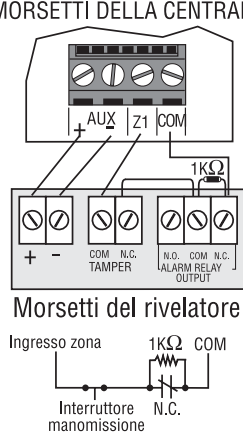
Contatti N.C., nessuna EOL Con riconoscimento manomissione MORSETTI DELLA CENTRALE
