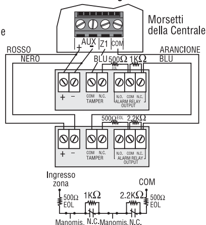
N.C., Nessuna EOL, con Riconoscimento manomissione e guasto cavo
