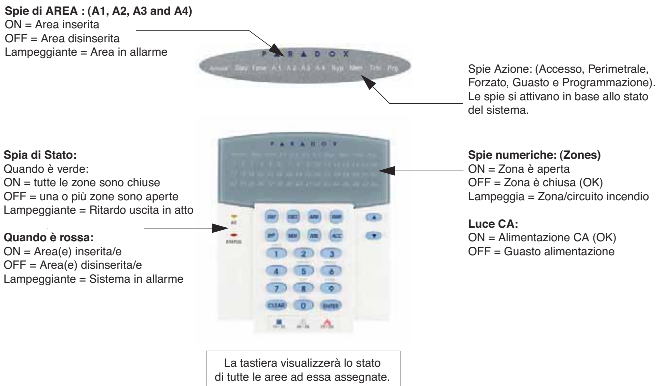
Figura 2: Panoramica tastiera a LED K648
