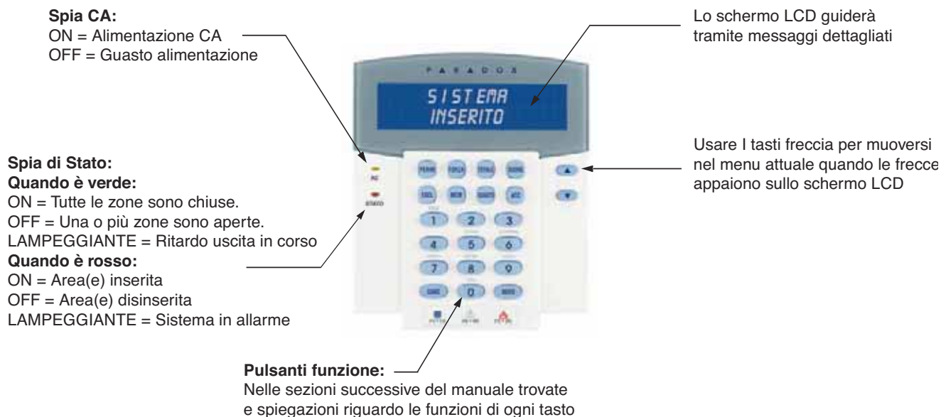
Figura 1: Panoramica di base della K641TIT/R
