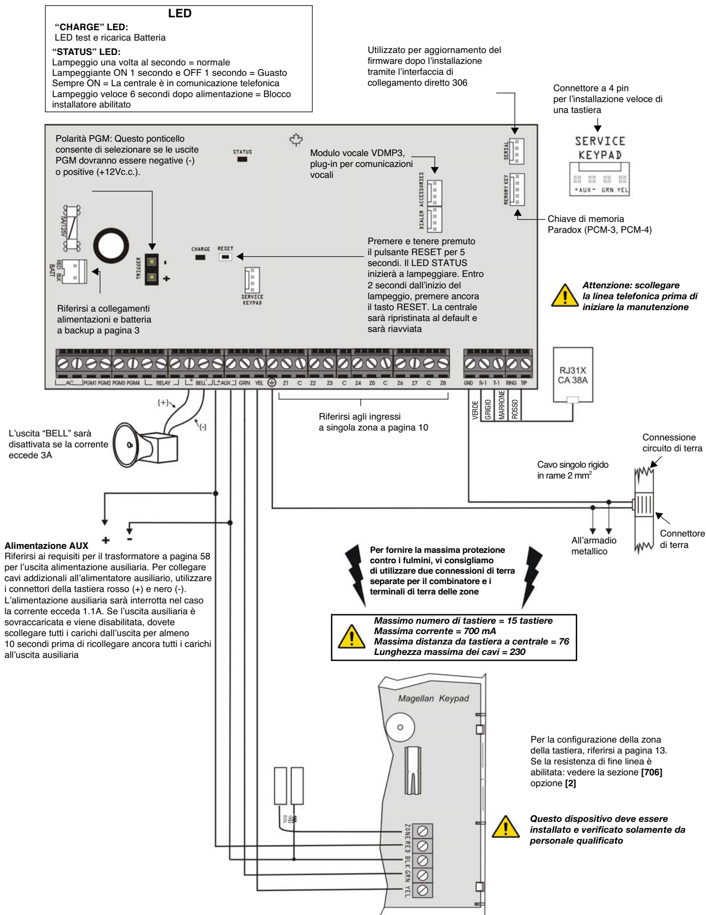
Fig. 5 - Descrizione scheda SP6000
