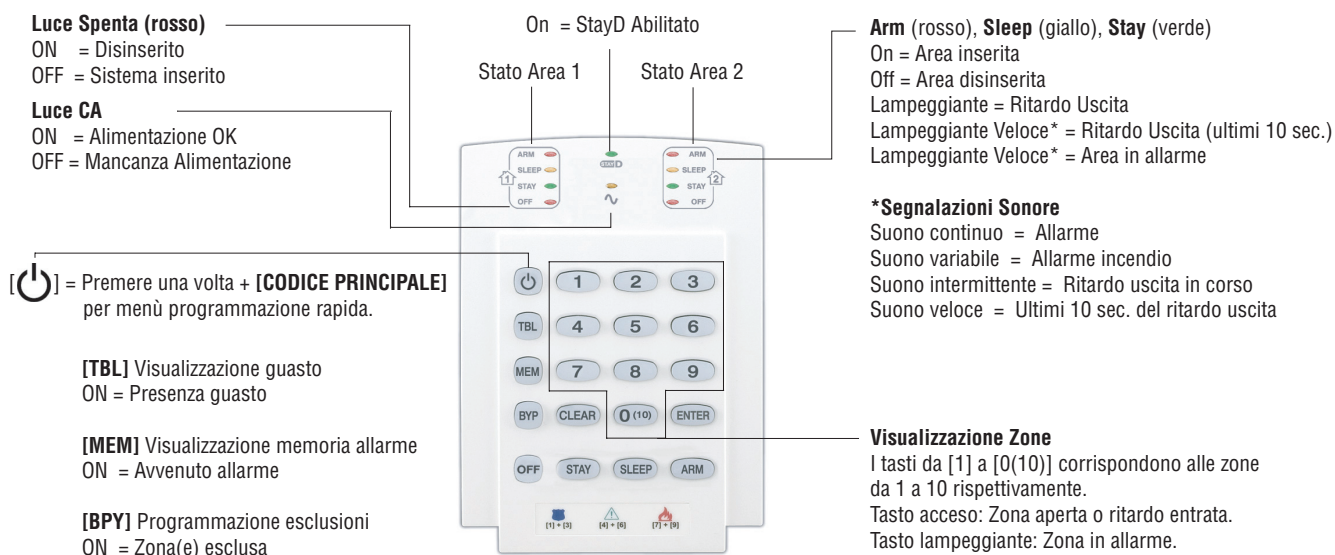
Figura 1: MG10LEDV/H (Moduli Tastiera 10 zone)
