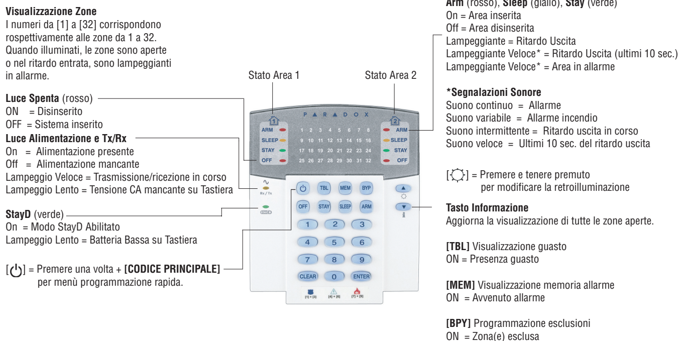
Figura 3 : MG32LRF (Modulo Tastiera Radio a 32 zone)
