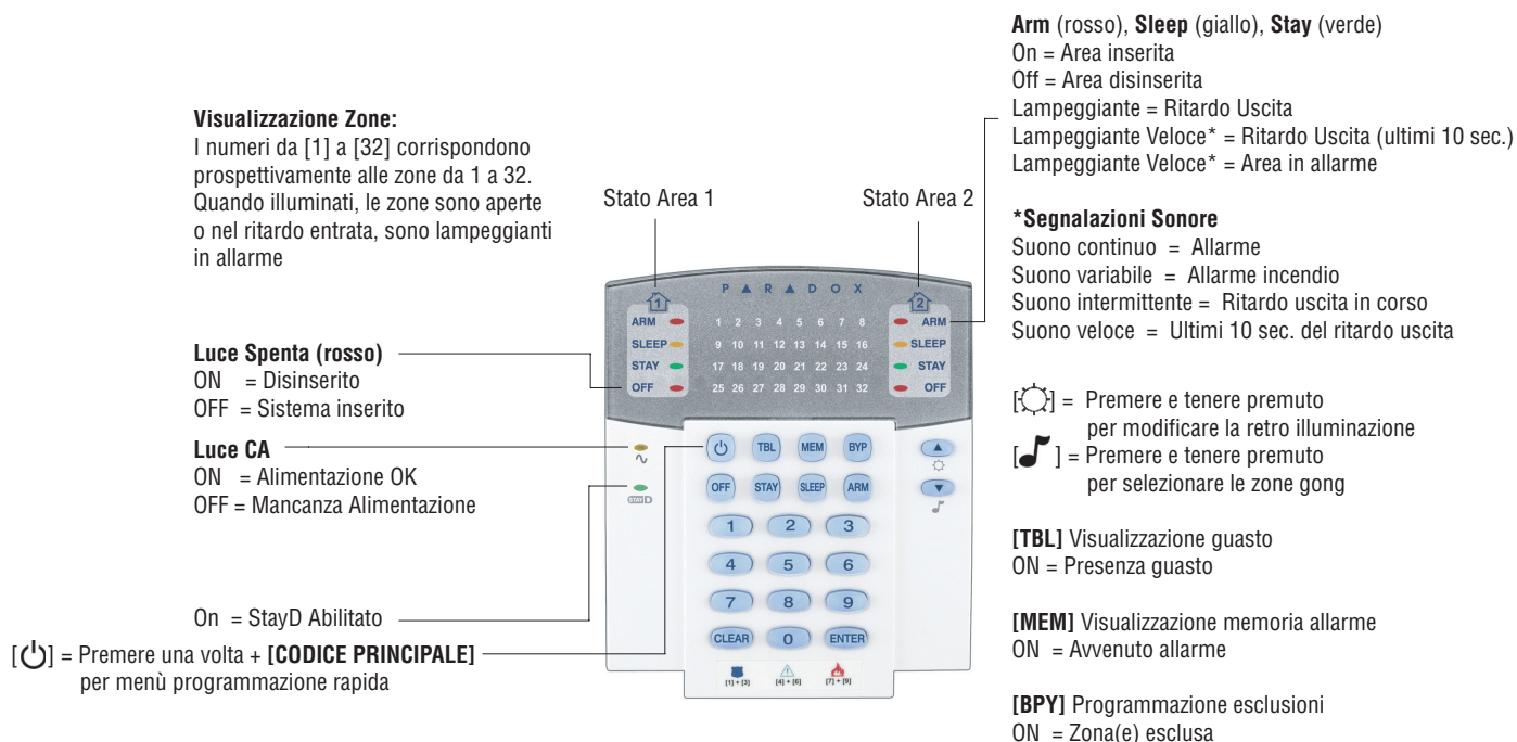
Figura 2 : MG32LED (Modulo Tastiera a 32 zone)
