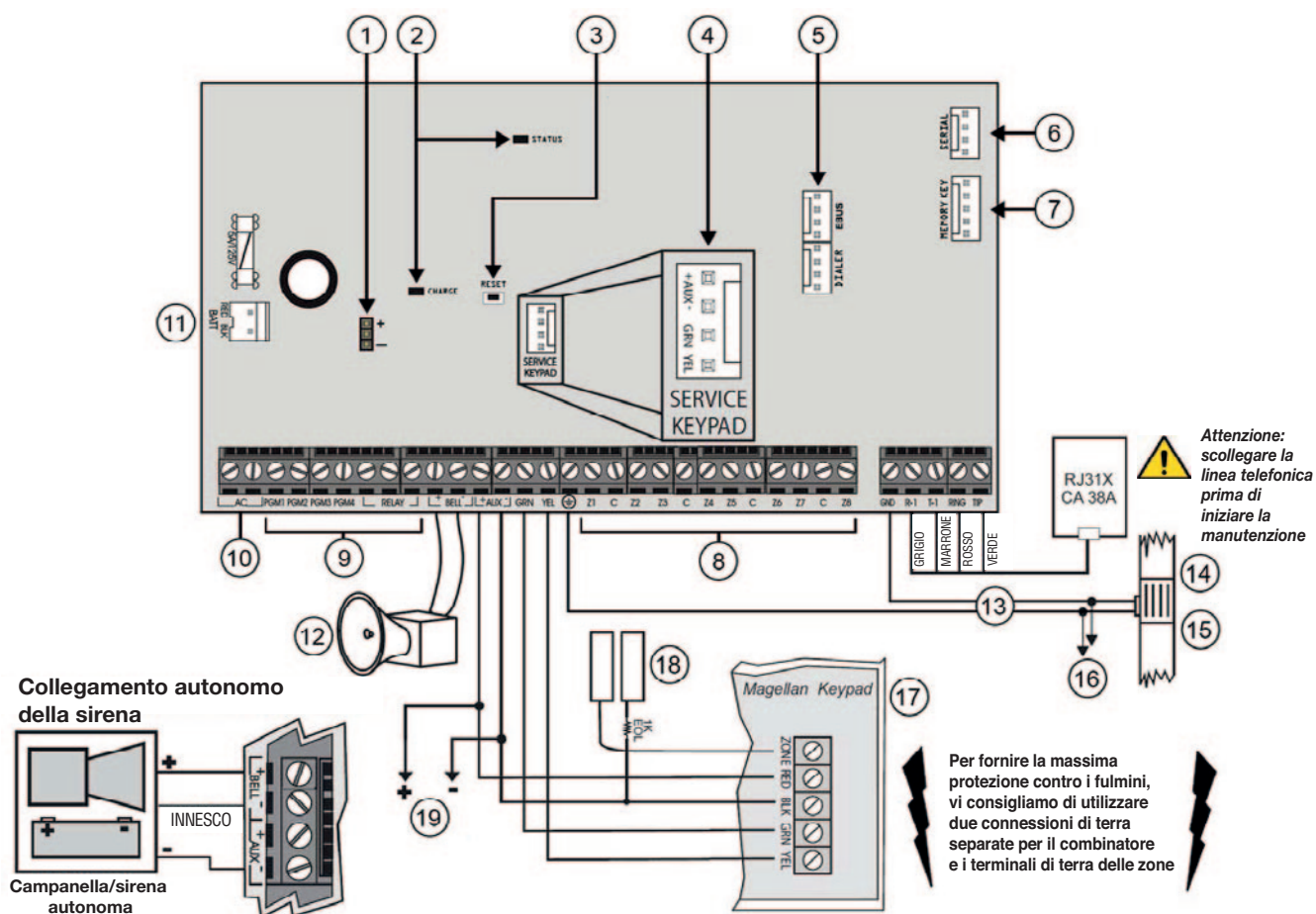
Fig. 7 - Descrizione scheda SP6000
