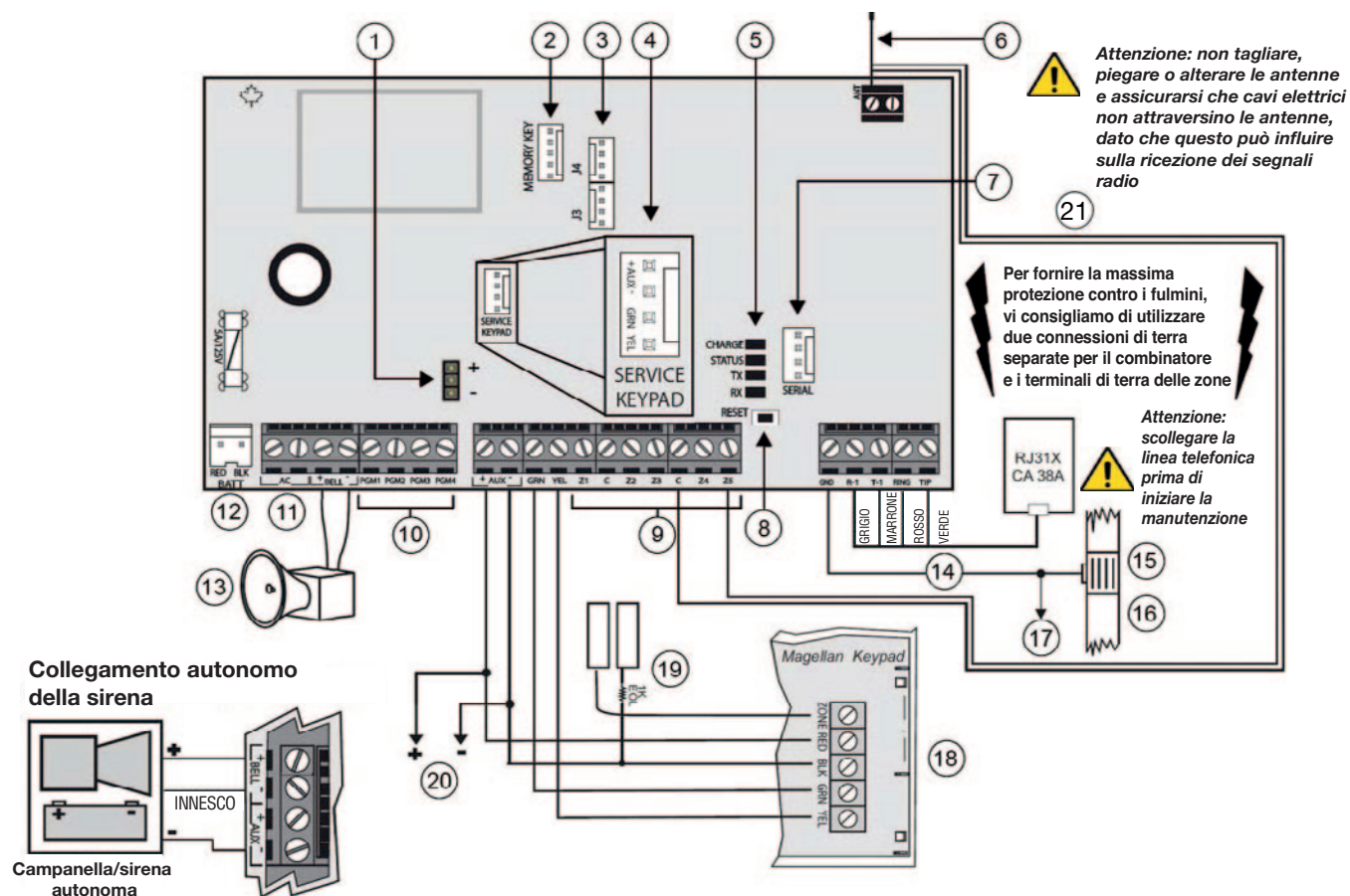
Fig. 3 - Descrizione scheda MG5050
