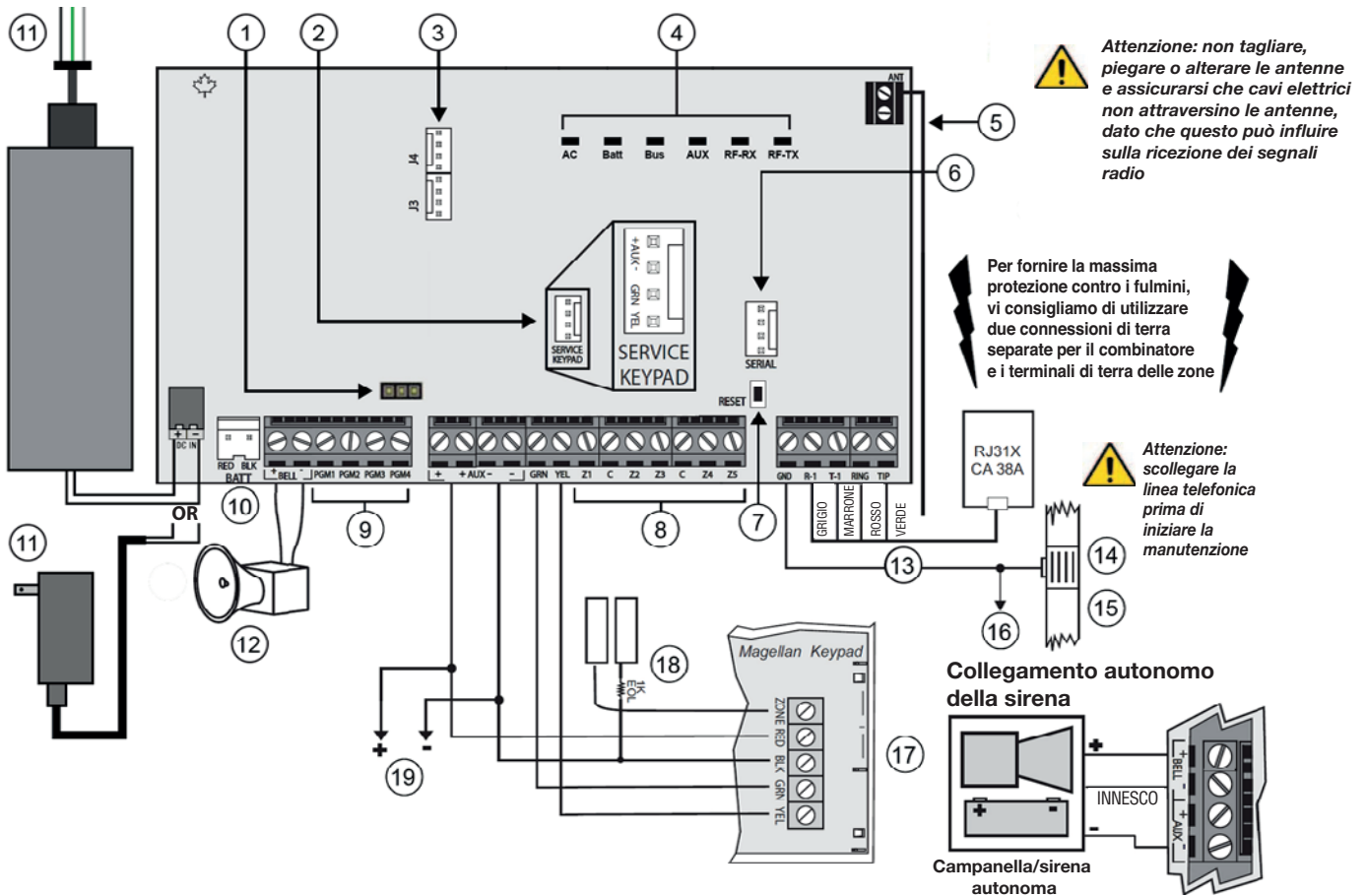
Fig. 4 - Descrizione scheda MG5075
