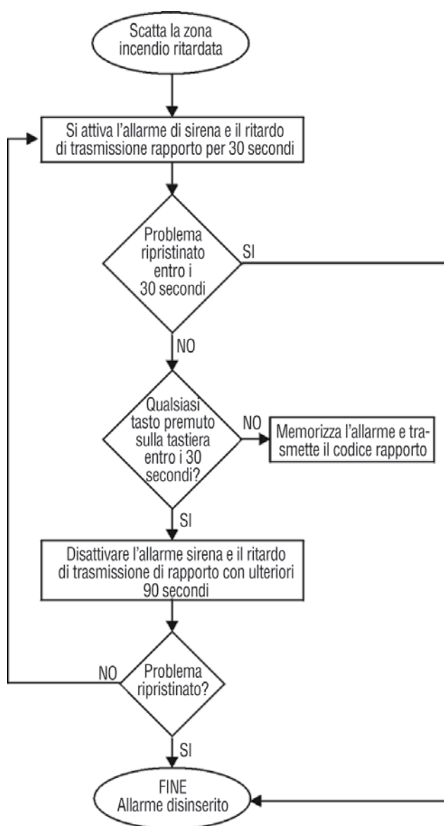
Fig 10 Zone incendio ritardate 24 ore
