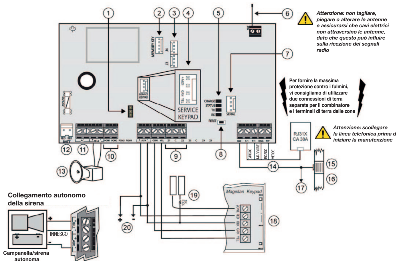
Fig. 2 - Descrizione scheda MG5000
