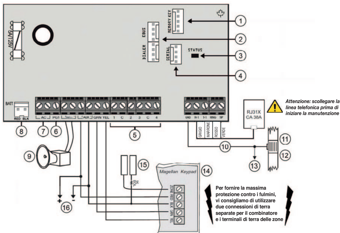
Fig. 5 - Descrizione scheda SP4000
