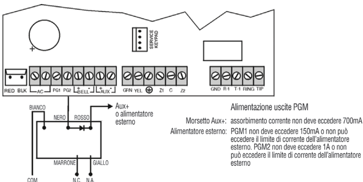
Fig. 7 - Collegamenti relé e PGM
