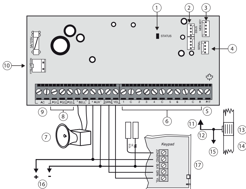
Fig. 8 - Descrizione scheda SP65
