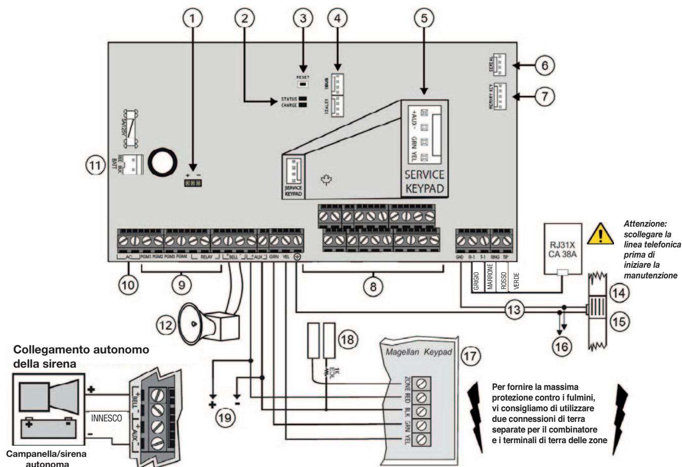
Fig. 9 - Descrizione scheda SP7000
