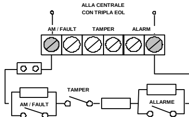
Schema di collegamento delle resistenze EOL
