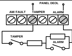
Schéma des résistances de fin de ligne
