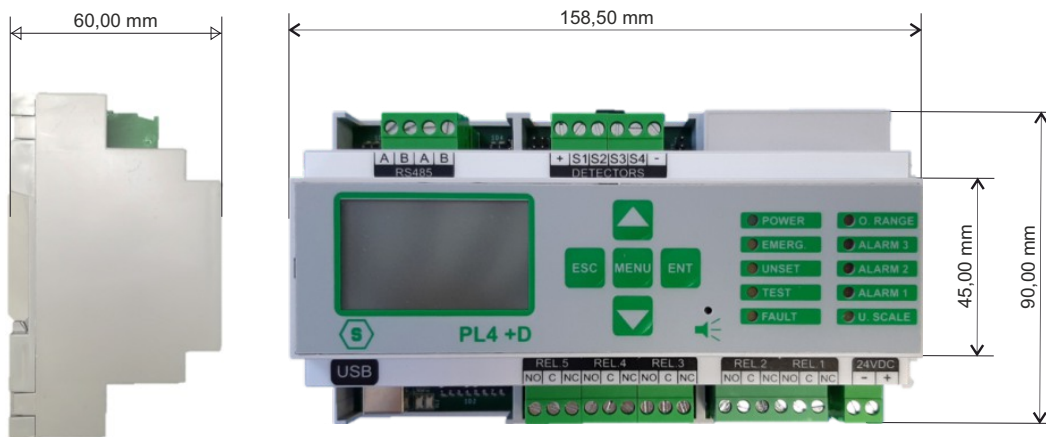
Figura 1) Vista centrale PL4+D con le relative quote
