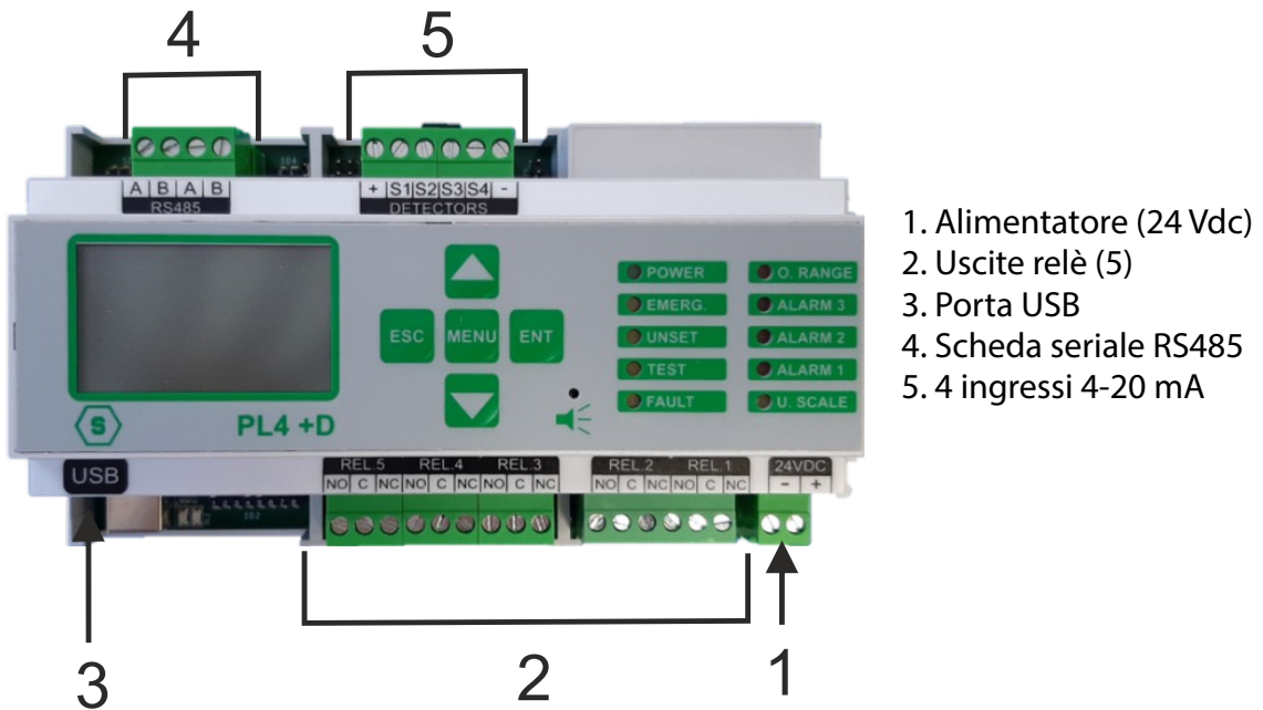
Figura 5) Identificazioni delle parti
