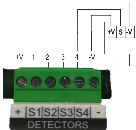
Figura 10) Collegamento dei 4 rilevatori in centrale
