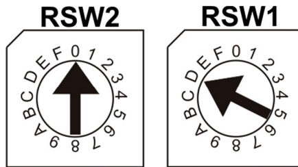
Figura 17) Esempio: se i due commutatori degli indirizzi sono impostati come sopra, RSW2 su 0 e RSW1 su D, l'indirizzo corrispondente in numeri decimali sarebbe 13 (vedere la tabella sotto).
