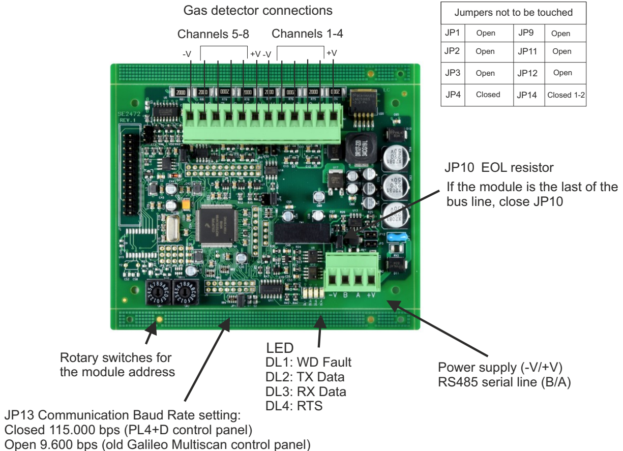
Figure 14) STG/IN8S module
