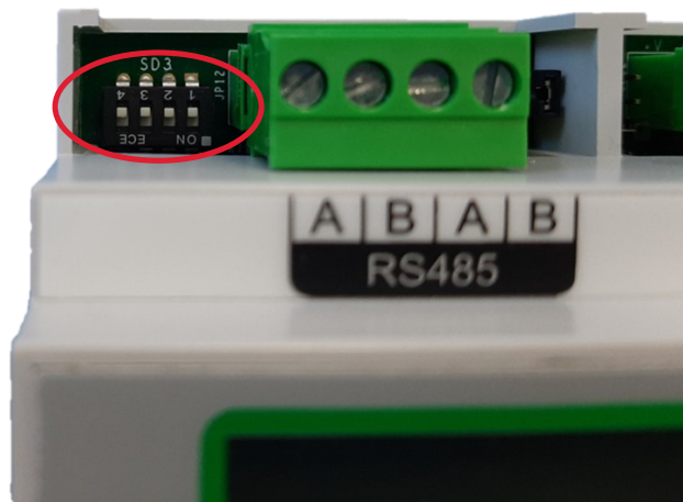
Figura 8) Serie di dip switch per l'impostazione della lingua
