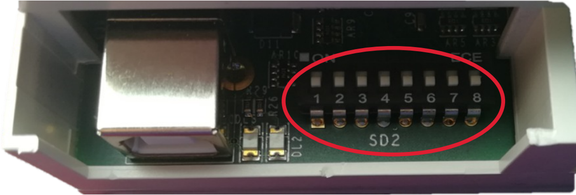
Figura 7) Serie di dip switch per impostazione baud rate
