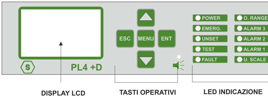
Figura 19) Pannello frontale centrale
