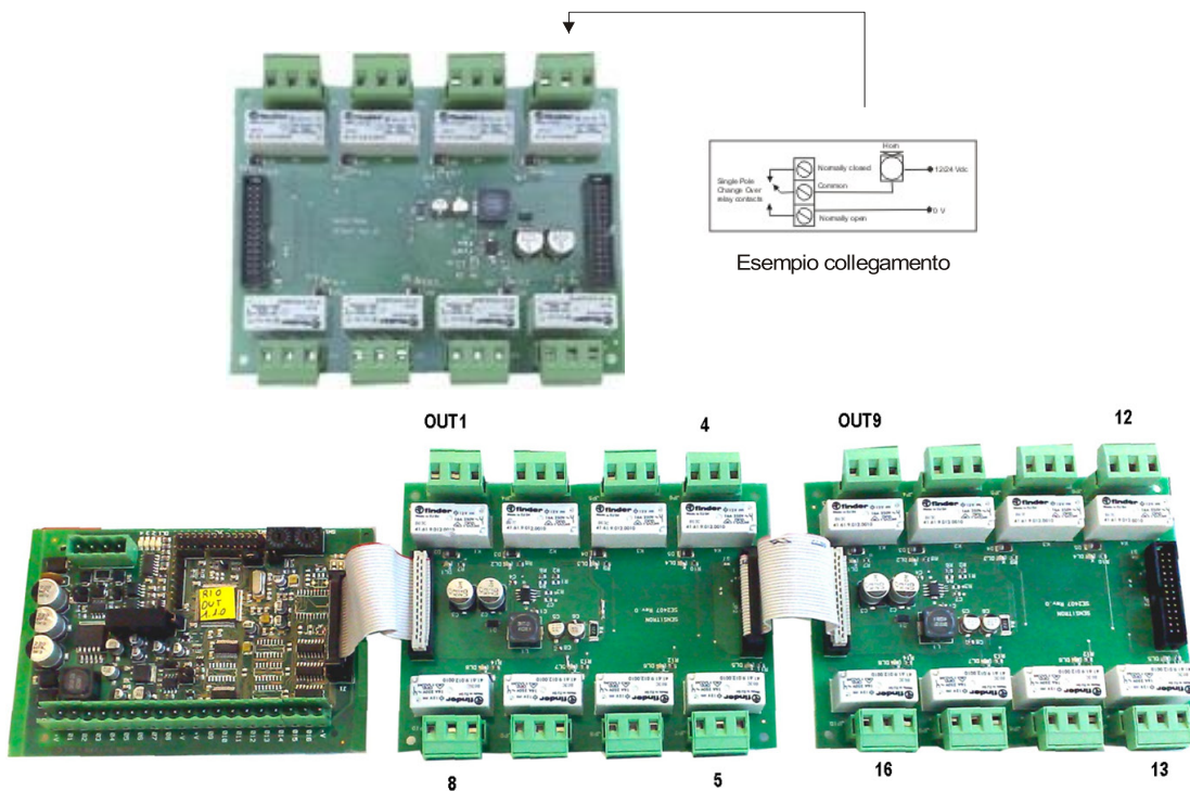
Figura 16) Scheda relè e collegamento a modulo uscita
