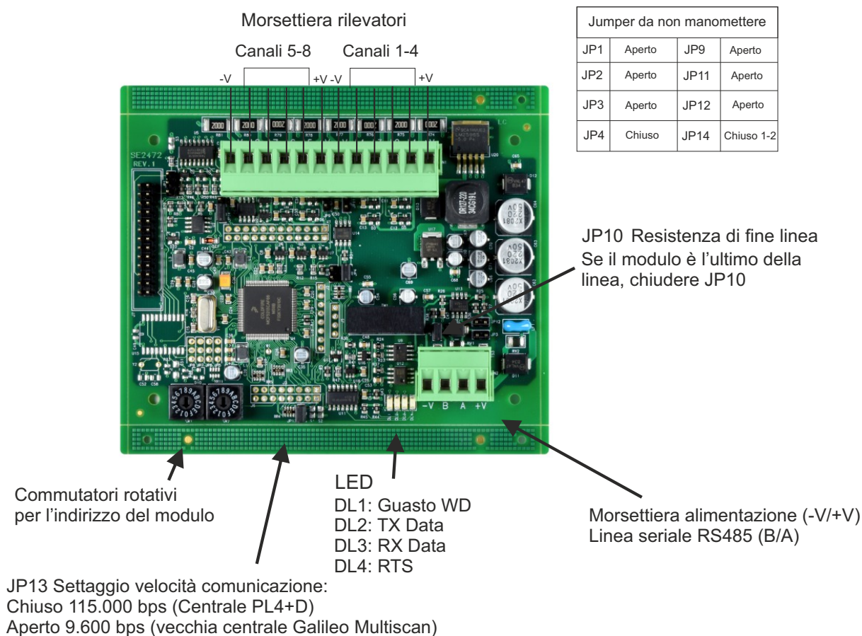
Figura 14) Modulo STG/IN8S
