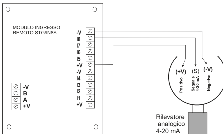
Figura 11) Collegamento degli 8 rilevatori al modulo STG/IN8S
