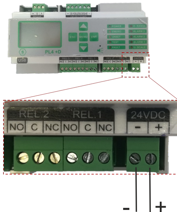
Figura 4) Collegamento cavo di alimentazione
