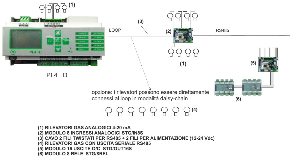
Figura 2) Schema a blocchi del sistema
