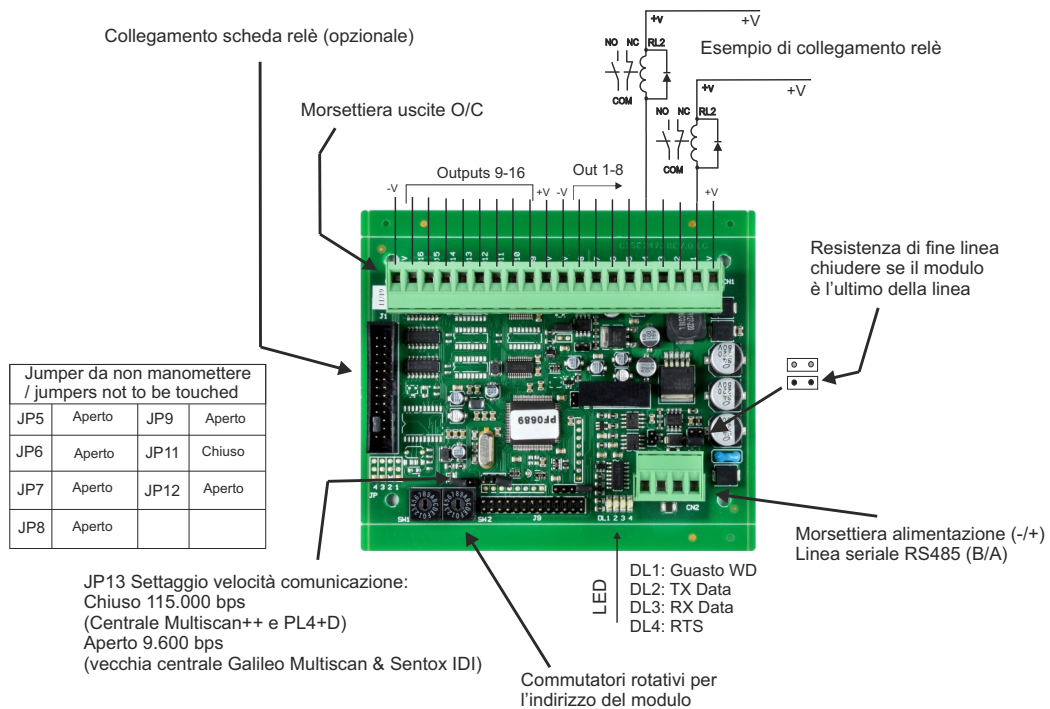
Figura 15) Modulo STG/OUT16S
