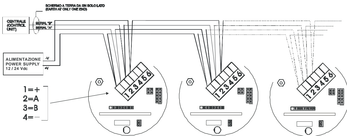
Esempio di collegamento rivelatori SMART3 NC su bus RS485 Example of connection of SMART3 NC detectors to a RS485 bus line
