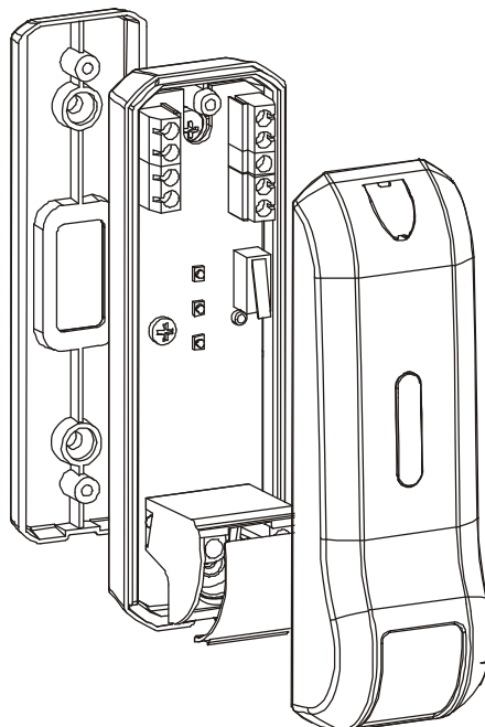
FISSAGGIO A PARETE
